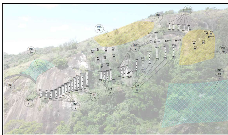
Figura 3: Identificação das Intervenções de Contenções de Encostas, localizadas no Bairro Comdusa, Vitória/ES. Fonte: Projeto Geotécnico prancha 02/18.
