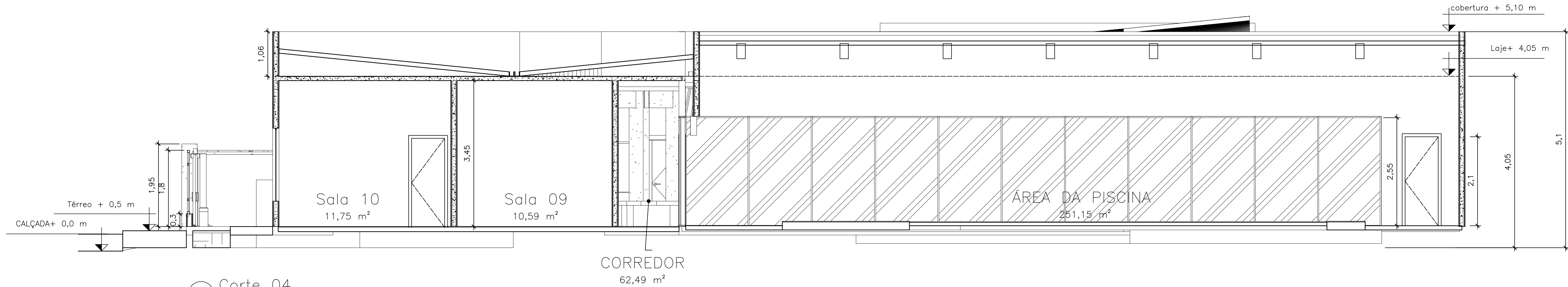
Corte 04 ESCALA 1/50
