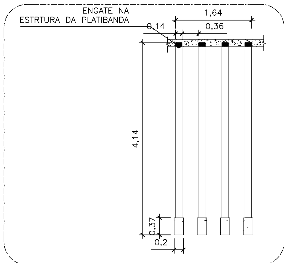
DET PERGOLADO 02 ESCALA 1/50
