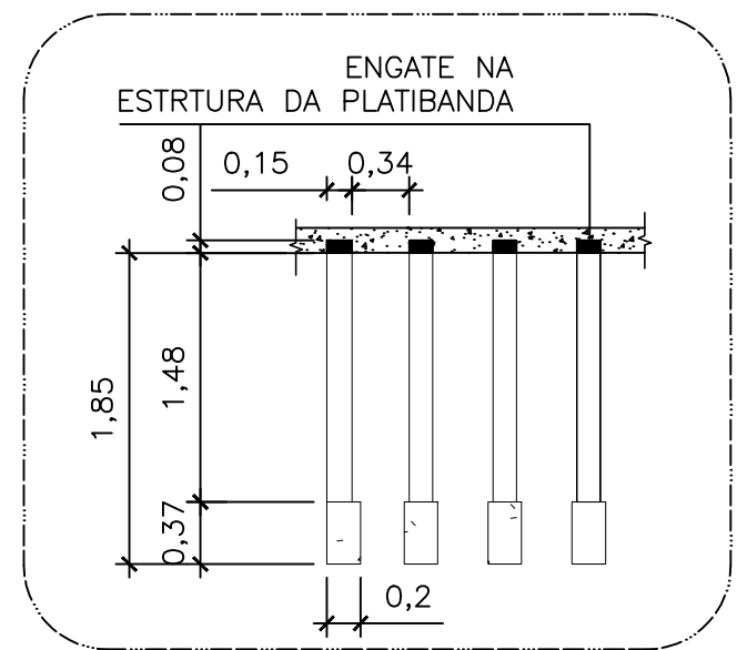
DET PERGOLADO 01 ESCALA 1/50
