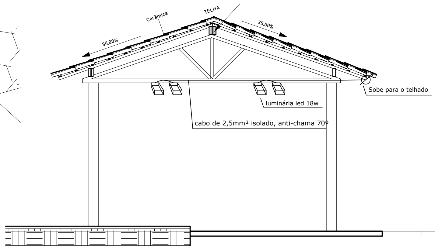
Corte 1
