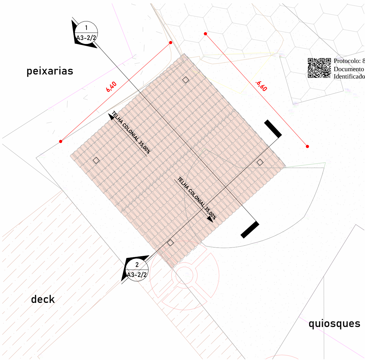
PÁV. SUPERIOR 1
