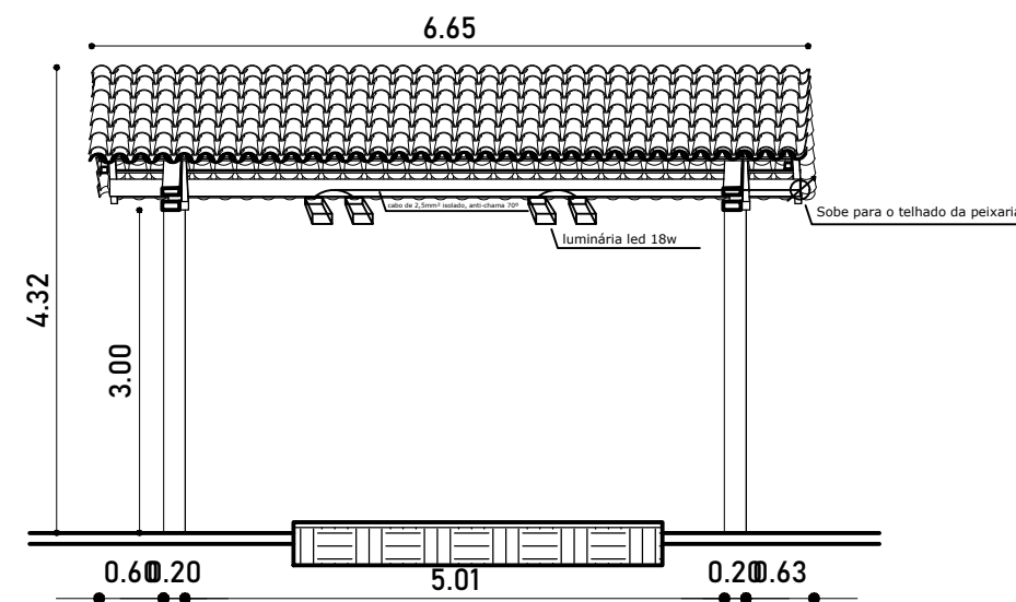
Corte 2
