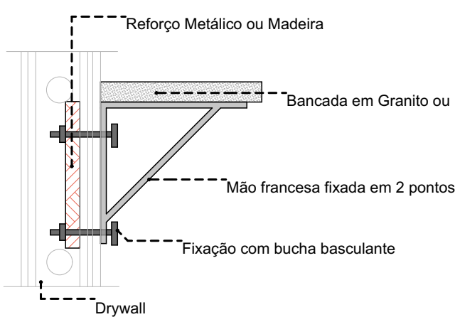
DETALHE 01: REFORÇO EM DRYWALL
