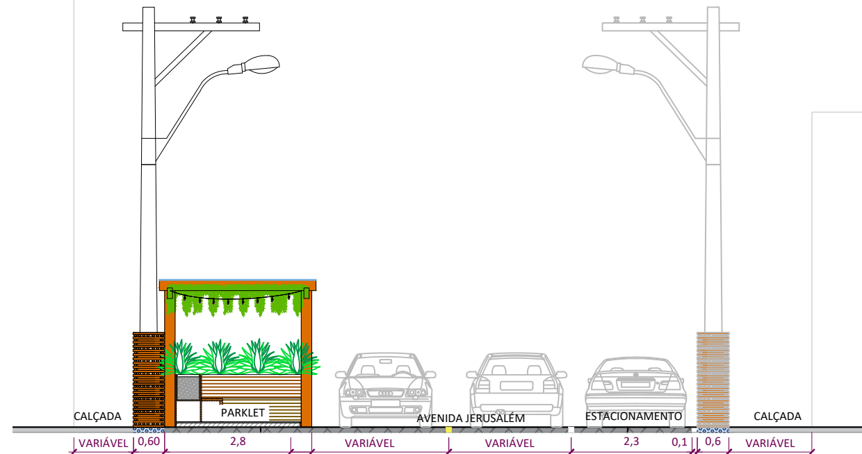
CORTE AA: AV. JERUSALÉM ESCALA 1/100
