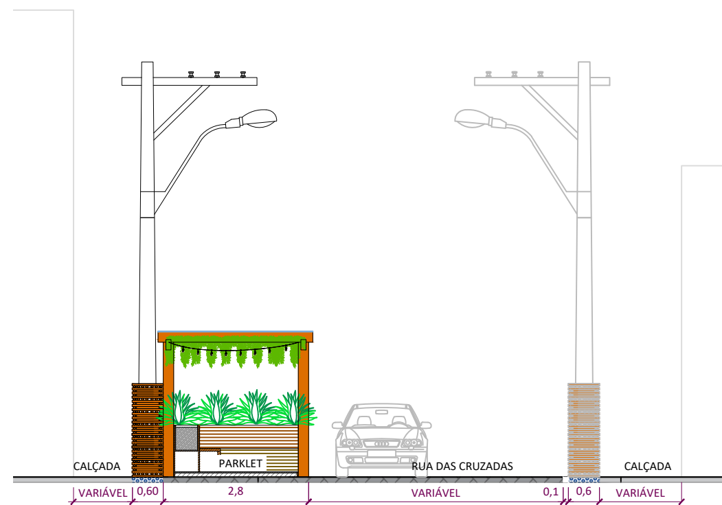
CORTE BB: RUA DAS CRUZADAS ESCALA 1/100
