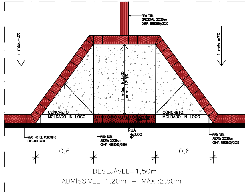
DET. 01 RAMPA DE ACESSO SEM ESCALA
