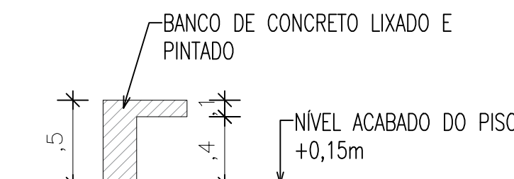
CORTE AA - BANCO CR. SEM ESCALA
