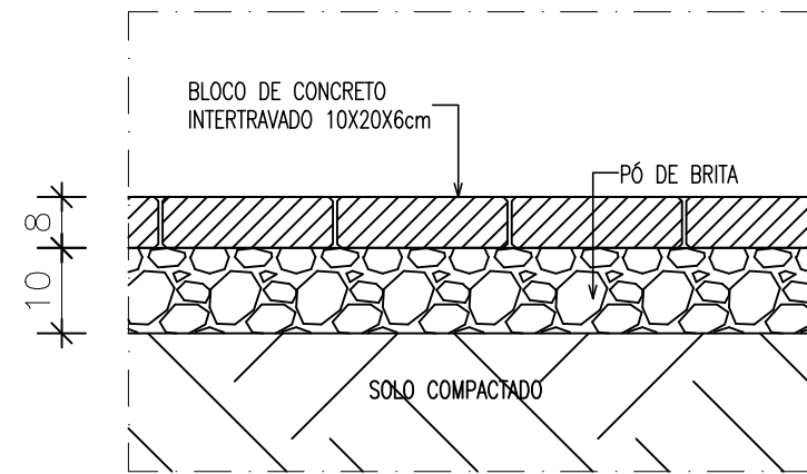
DET. PISO BLOCO INTERTRAVADO SEM ESCALA
