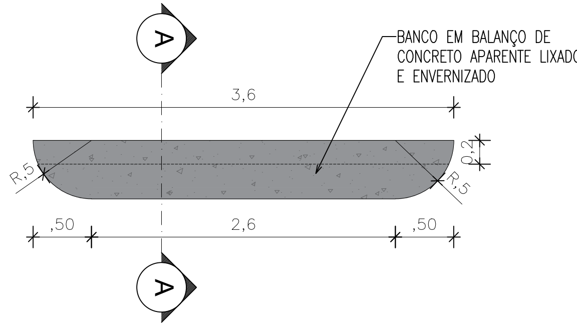
VISTA SUPERIOR BANCO CR. SEM ESCALA
