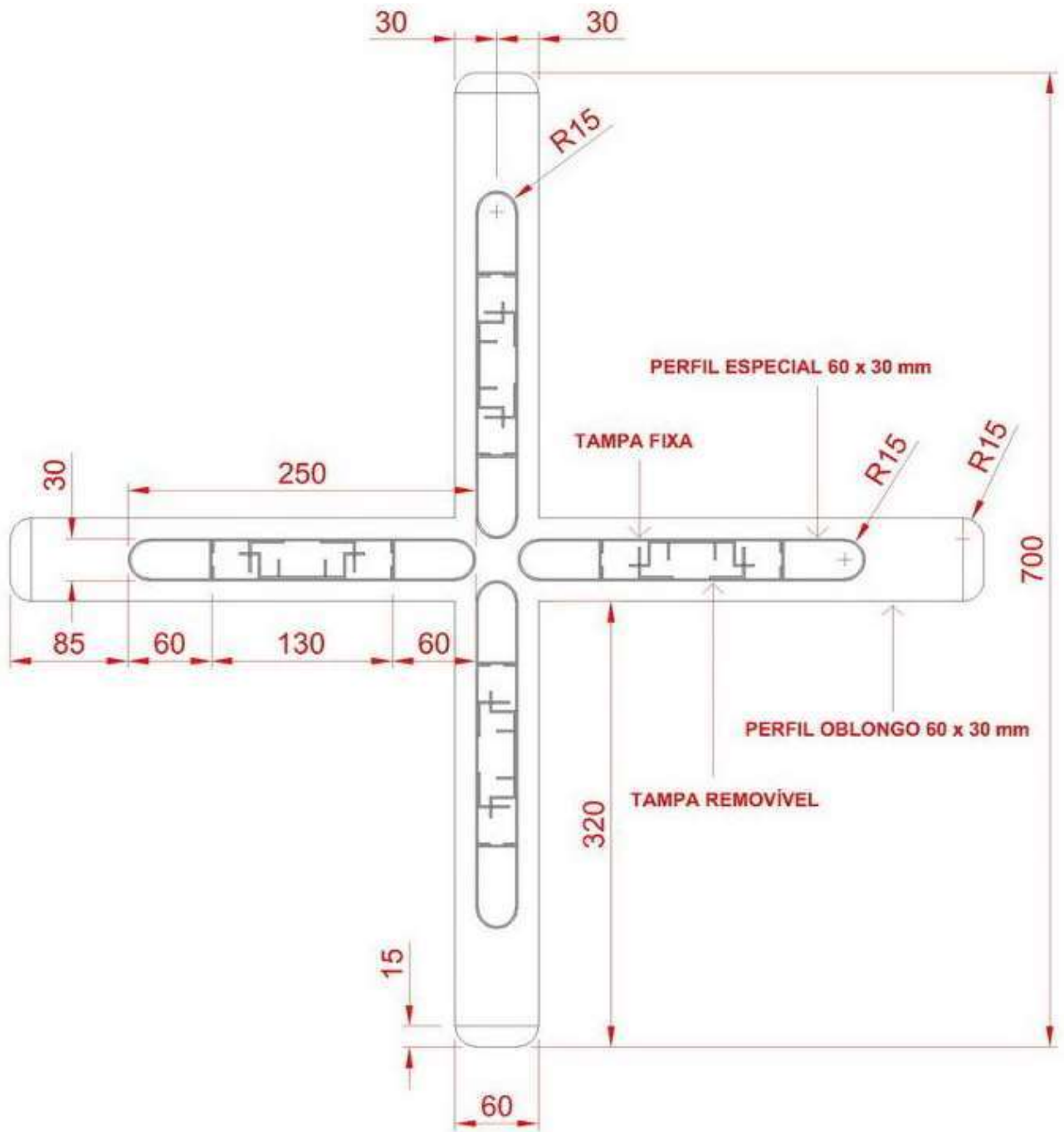
CORTE 'AA'
