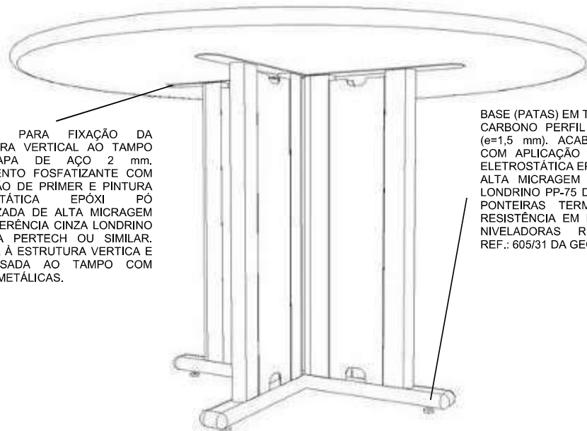
PERSPECTIVA 02
