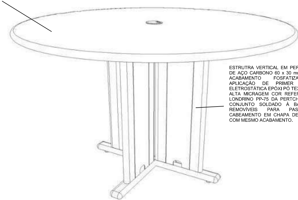
PERSPECTIVA 01
