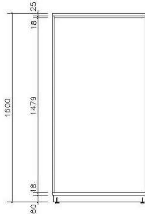
ELEVAÇÃO POSTERIOR ARMÁRIO ALTO - AA0 ao AA4 ESCALA 1:20
