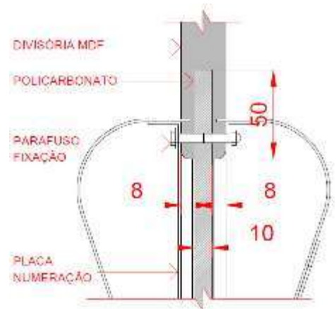
DETALHE ENCAIXE POLICARBONATO
