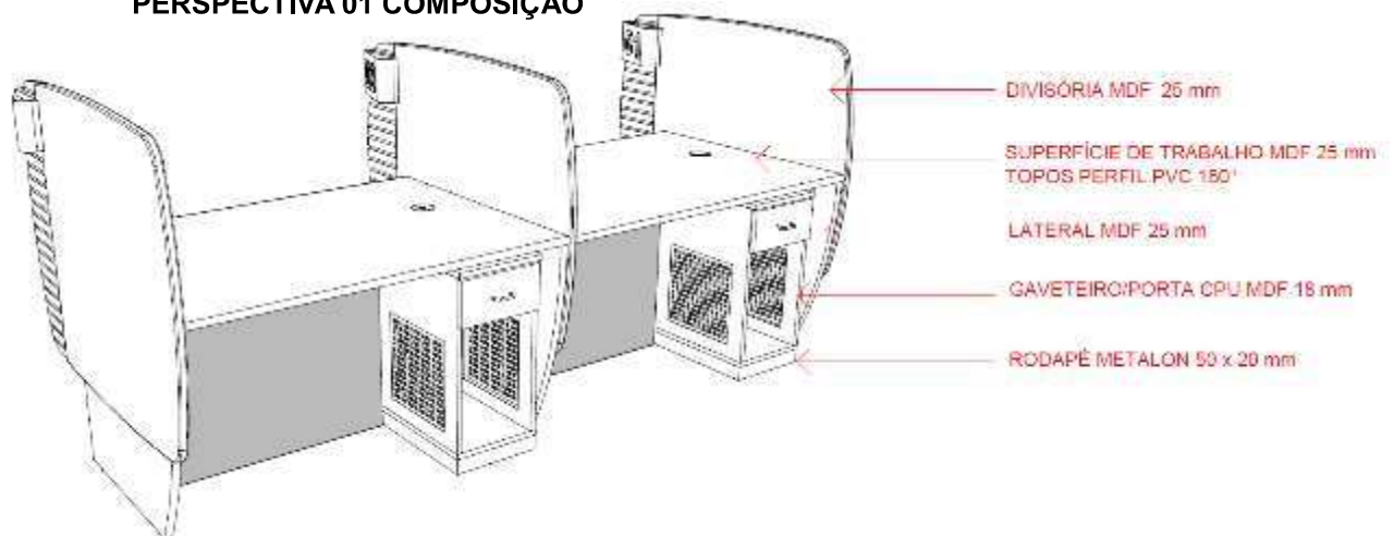
PERSPECTIVA 01 COMPOSIÇÃO
