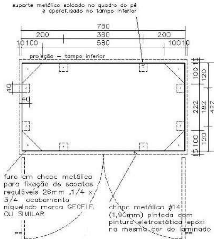
PLANTA BAIXA BASE METÁLICA ESCALA 1:10
