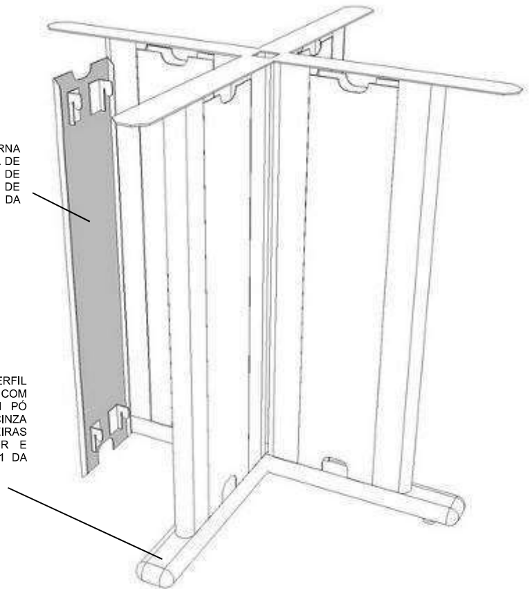
PERSPECTIVA 04
