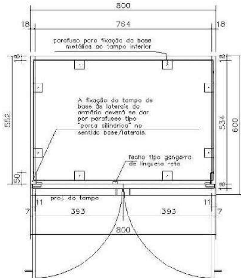
PLANTA BAIXA TAMPO INFERIOR ESCALA 1:10
