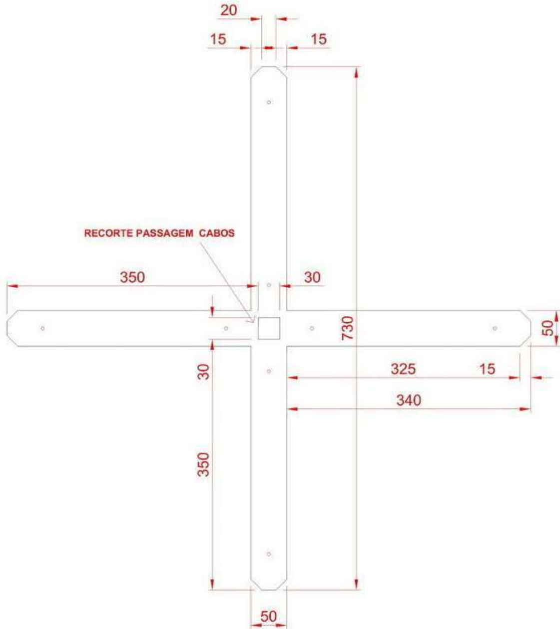
CRUZETA FIXAÇÃO ESTRUTURA/TAMPO
