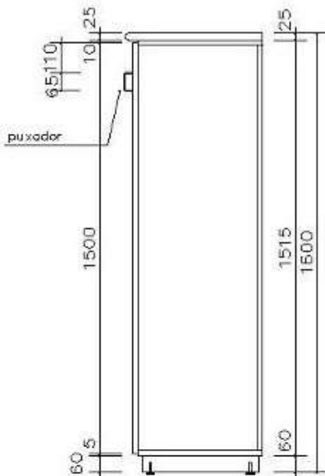
ELEVAÇÃO LATERAL ARMÁRIO ALTO - AA0 ao AA4 ESCALA 1:20
