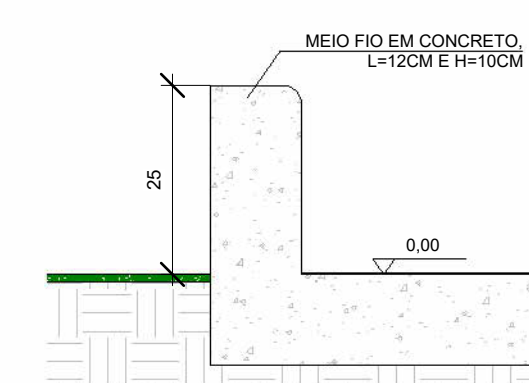
3 DET. MEIO-FIO (CANTEIROS) 1:50
