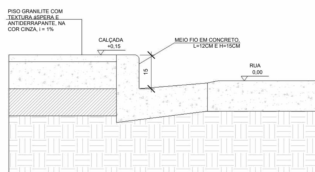
DETALHE MEIO-FIO (VIA) 1:50
