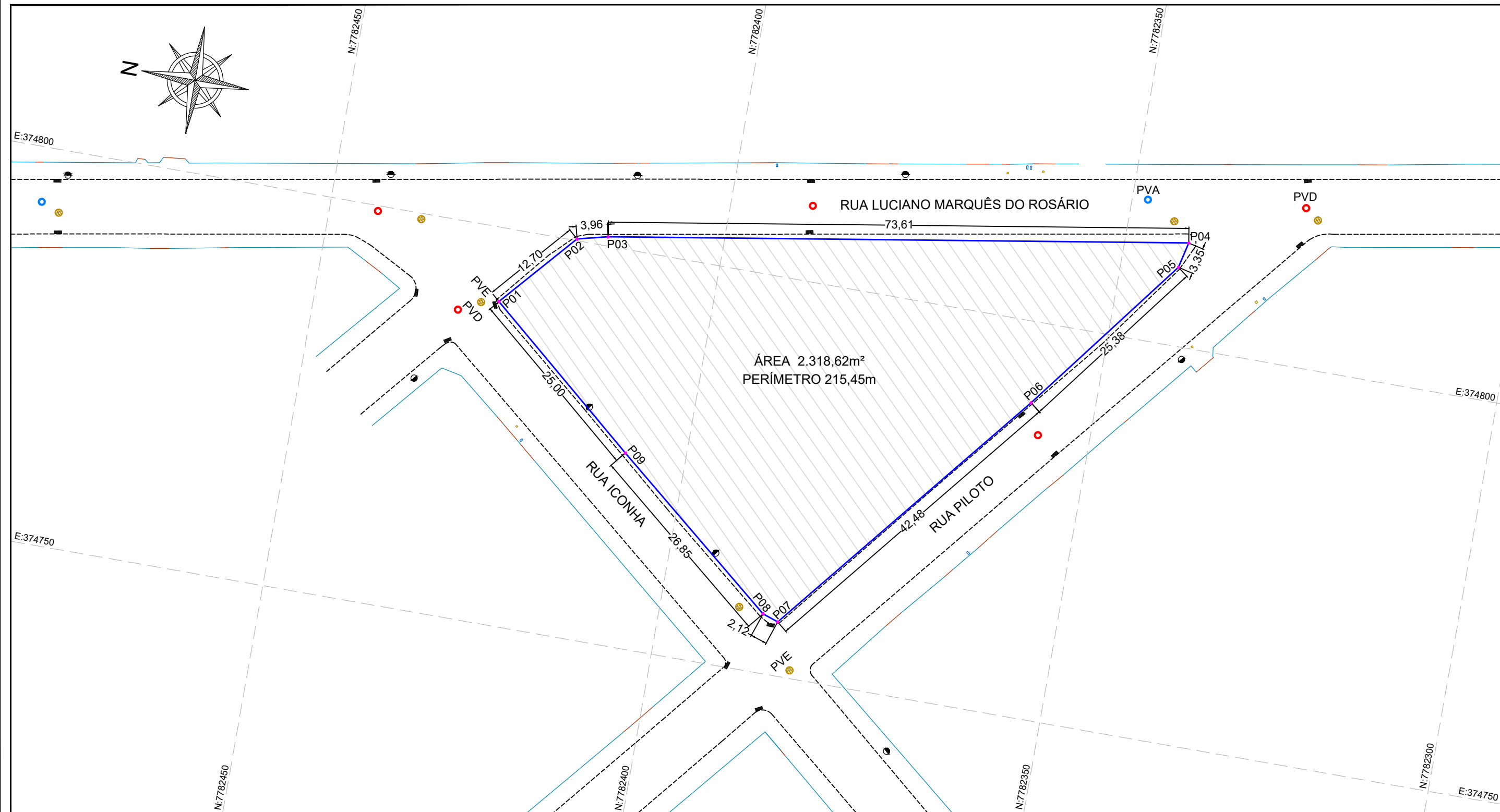
PLANTA DE SITUAÇÃO ESCALA 1:500
