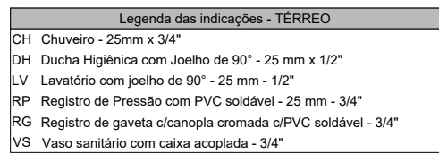
DETALHE HID-1 1:25
