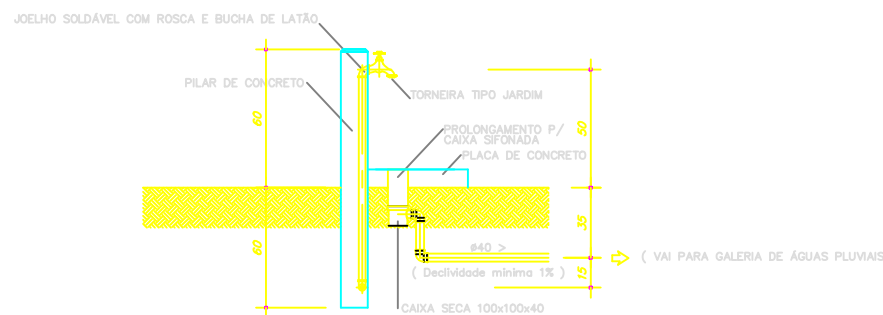
VISTA LATERAL PUNTO DE ÁGUA EXTERNO Sem Escala
