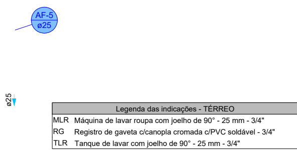
DETALHE HID-2 1:25
