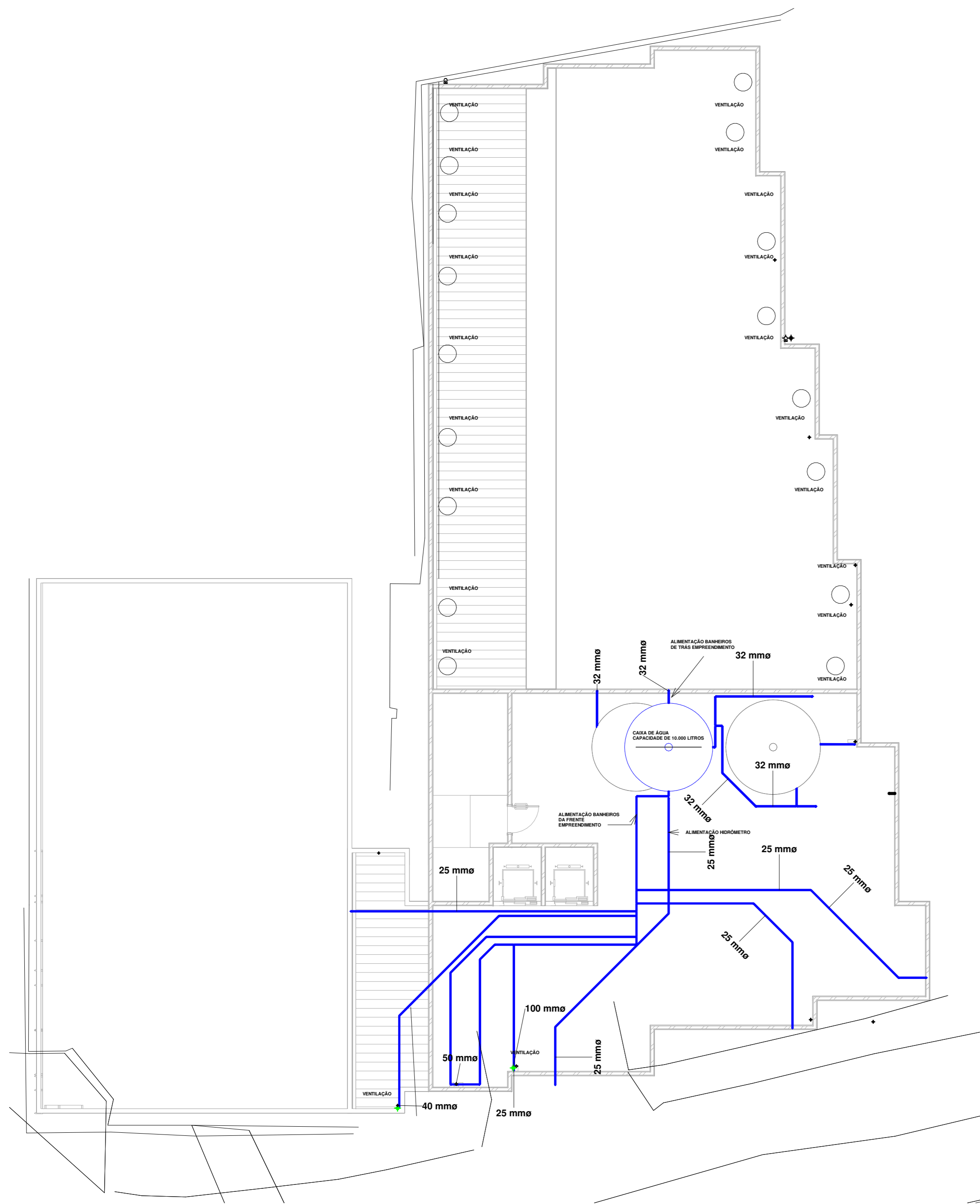
4 Planta baixa do 3º pavimento. 1:110
