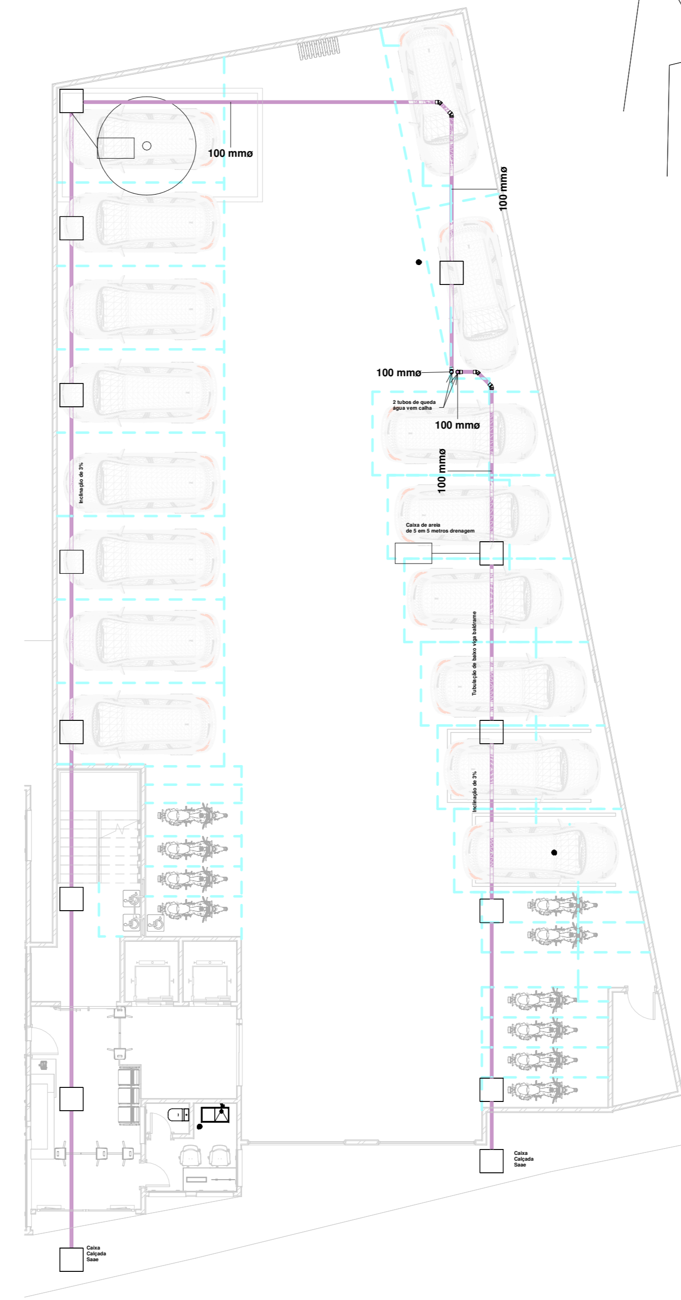
5 Planta baixa do térreo.AP. 1:110
