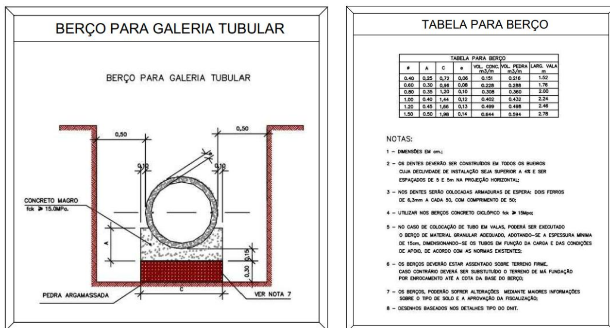
Figura 5: Detalhe de execução de berço para tubos de concreto
