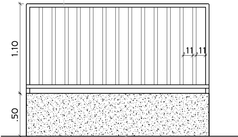
GUARDA CORPO FIXADO SOBRE MURO DE CONTENÇÃO A SER EXECUTADO
