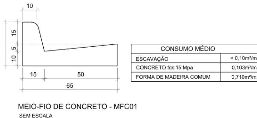
Figura 6: Detalhe do meio fio a ser utilizado
