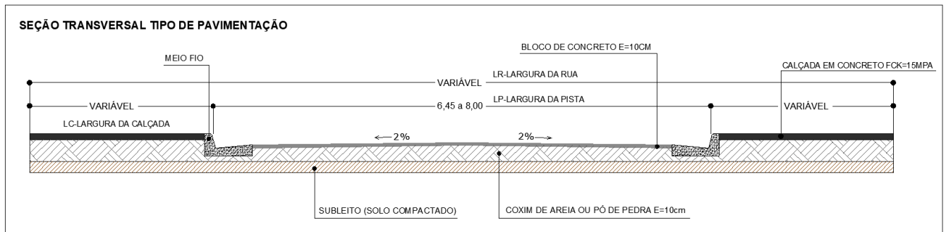
Figura 2: Detalhe tipo da pavimentação
