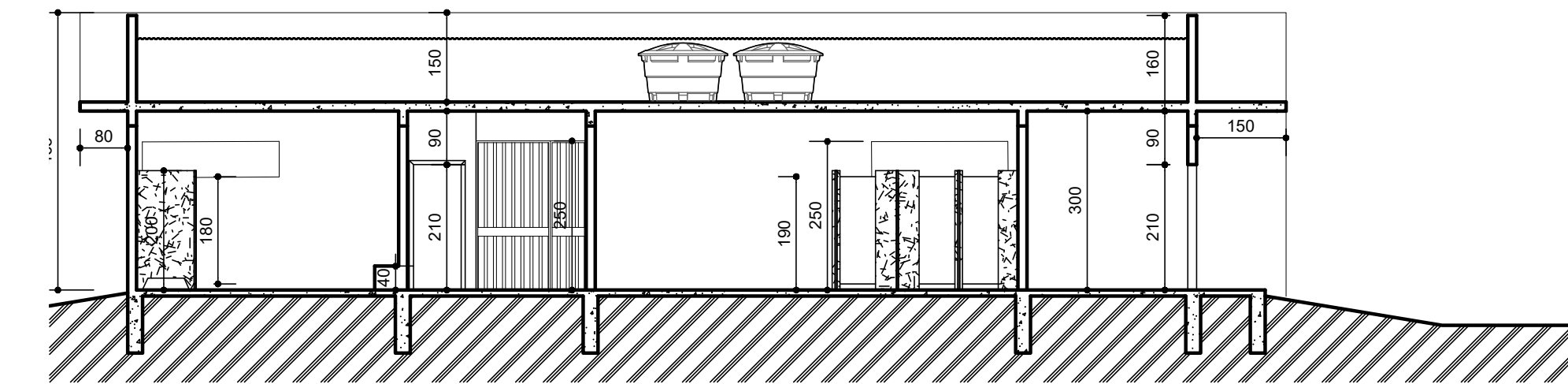
03 Corte AA Escala: 1:100
