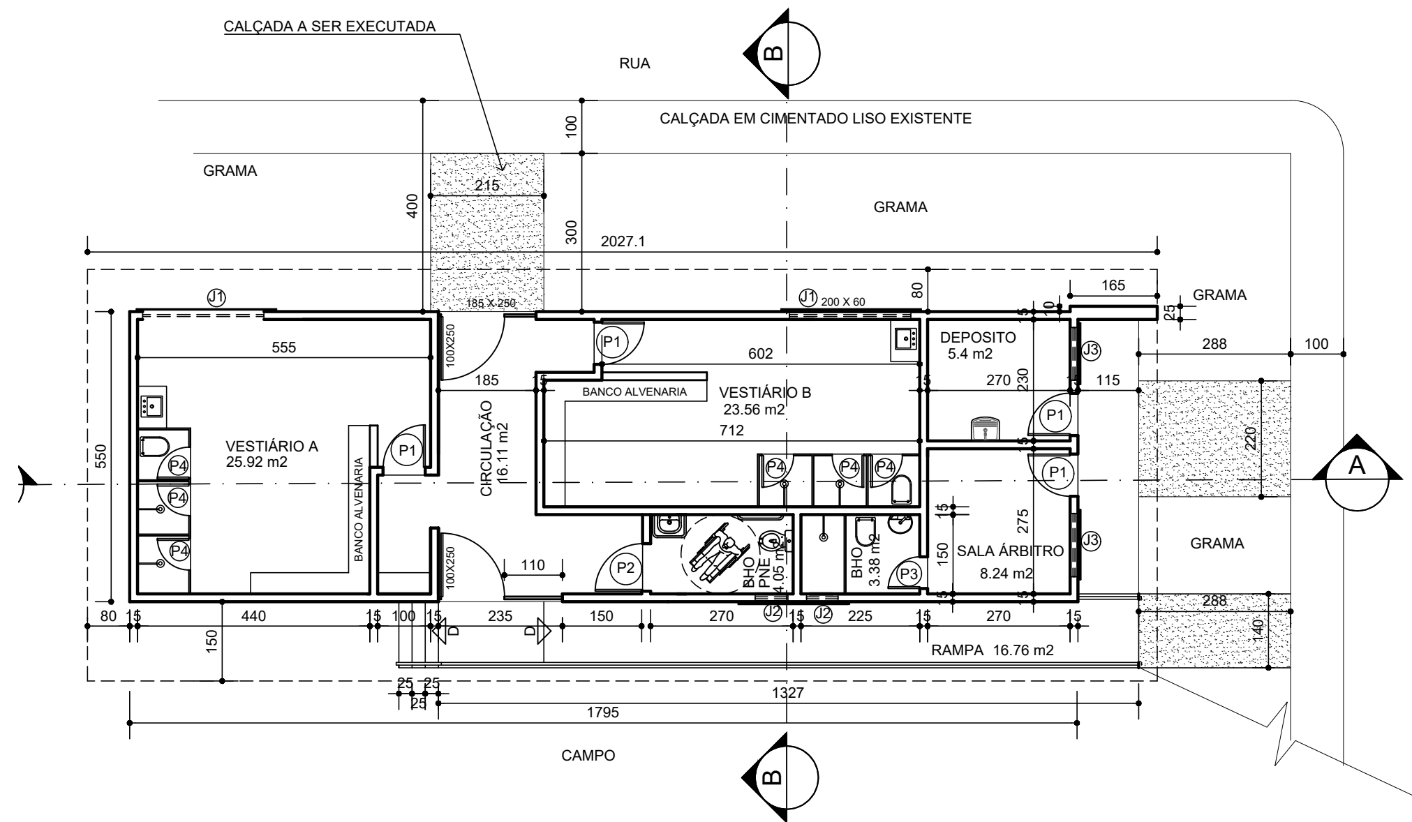
01 Planta Escala: 1:100
