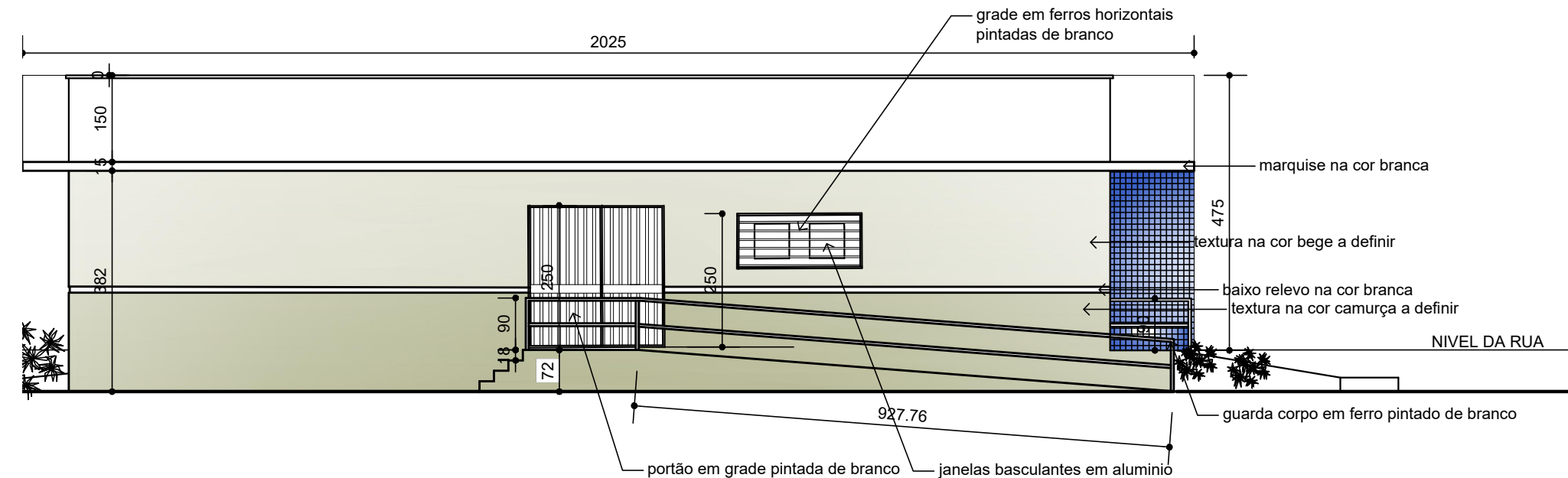
06 FACHADA PARA O CAMPO Escala: 1:100
