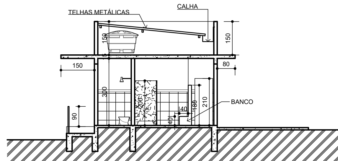
04 Corte BB Escala: 1:100
