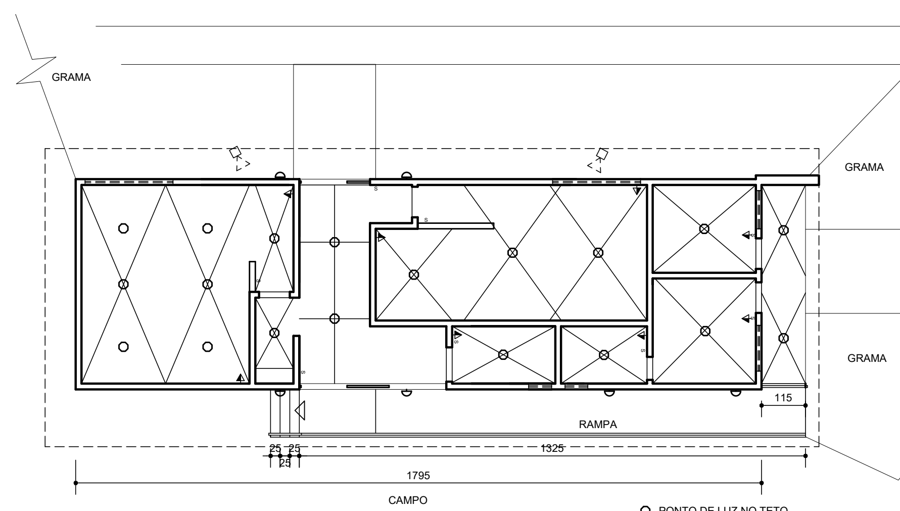
02 PONTOS DE LUZ Escala: 1:100
