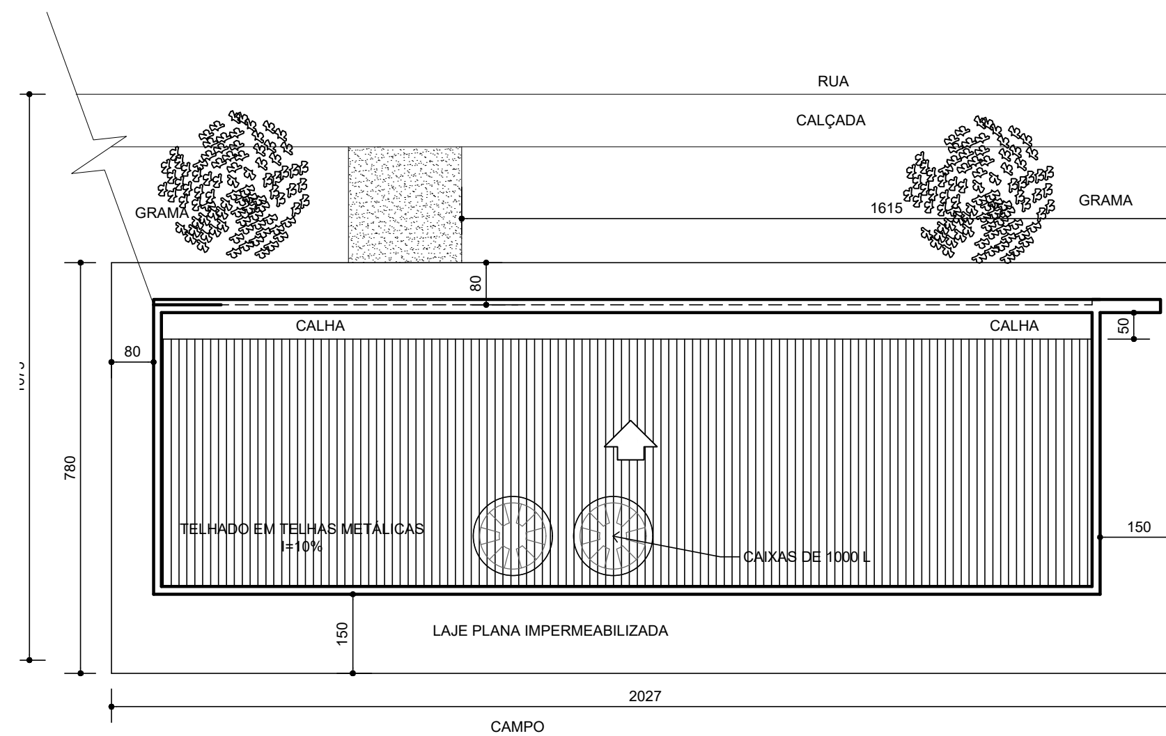
02 COBERTURA / SITUAÇÃO Escala: 1:100
