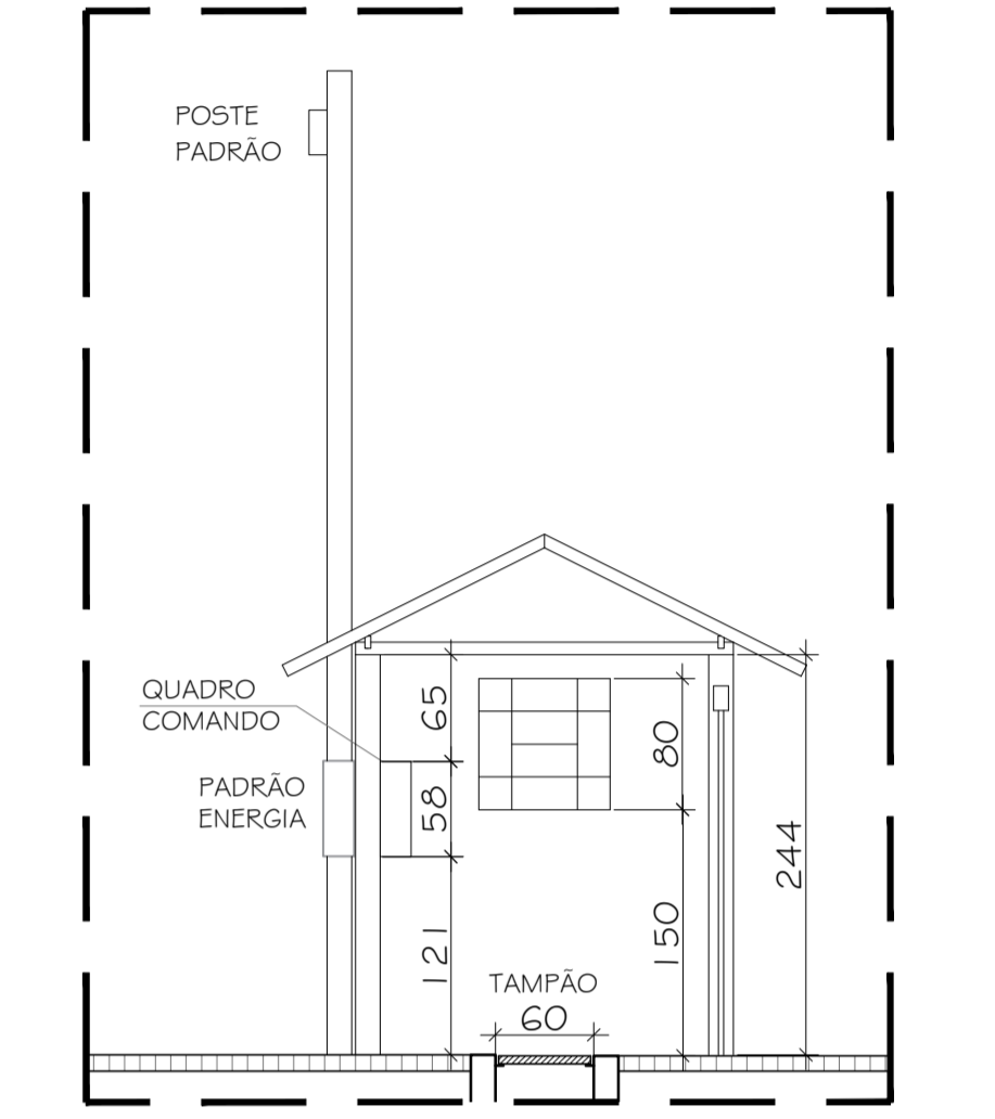
09 DETALHE D - CASA DE COMANDO ESCALA 1/50
