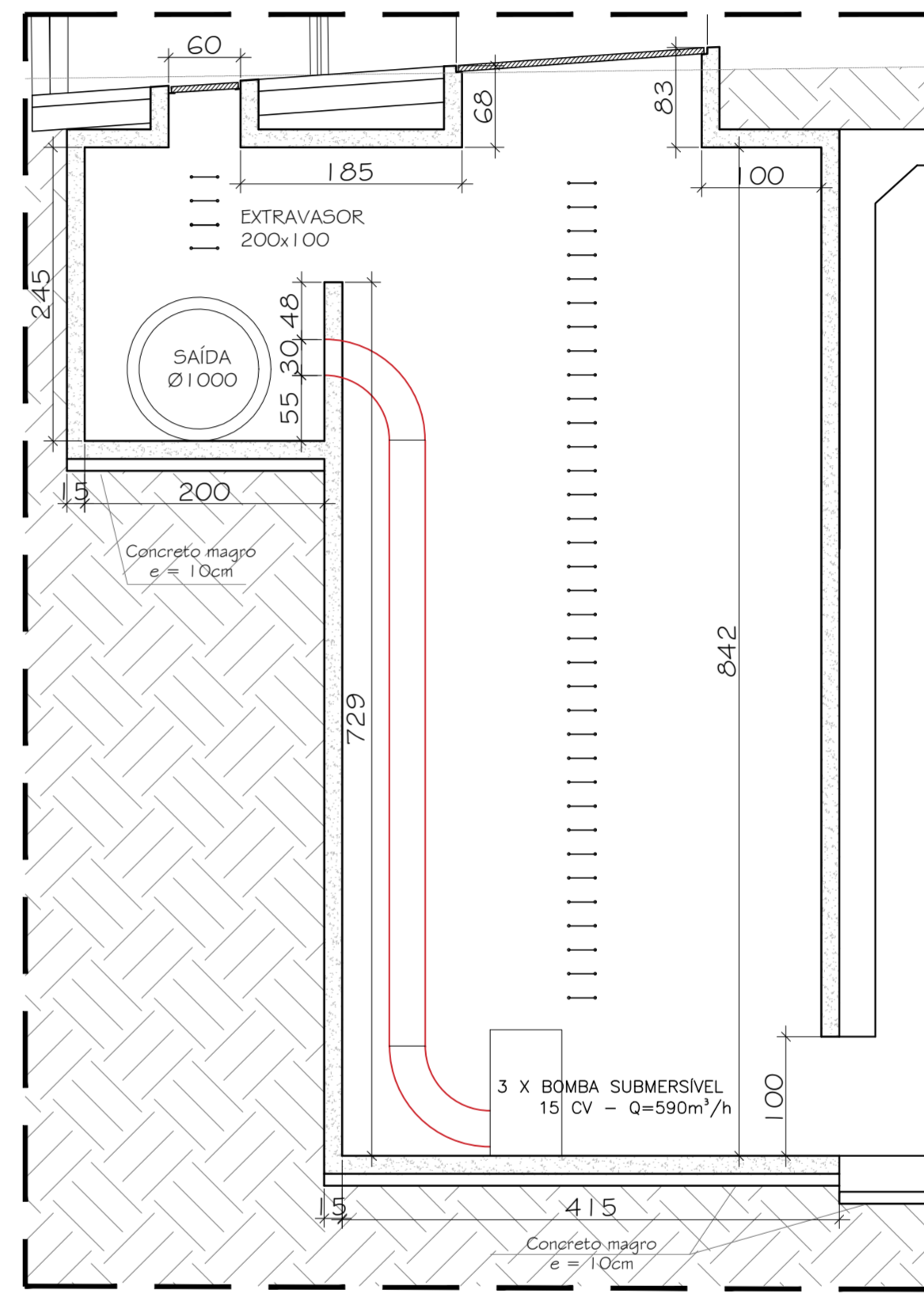
07 DETALHE B - CAIXA DE SAÍDA ESCALA 1/50
