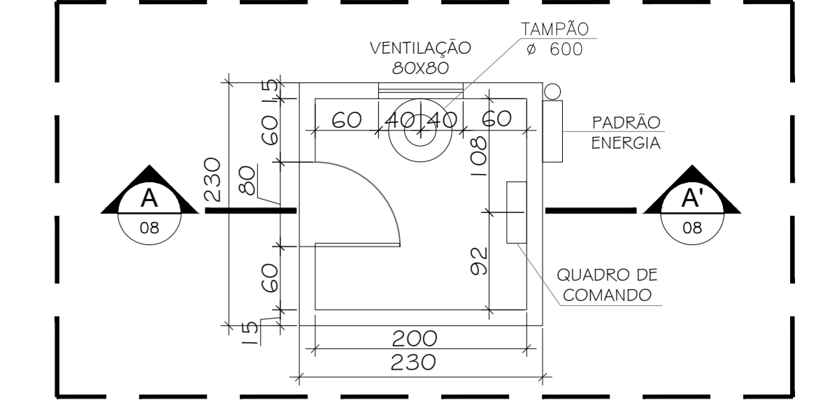
08 DETALHE D - PLANTA BAIXA CASA DE COMANDO ESCALA 1/50
