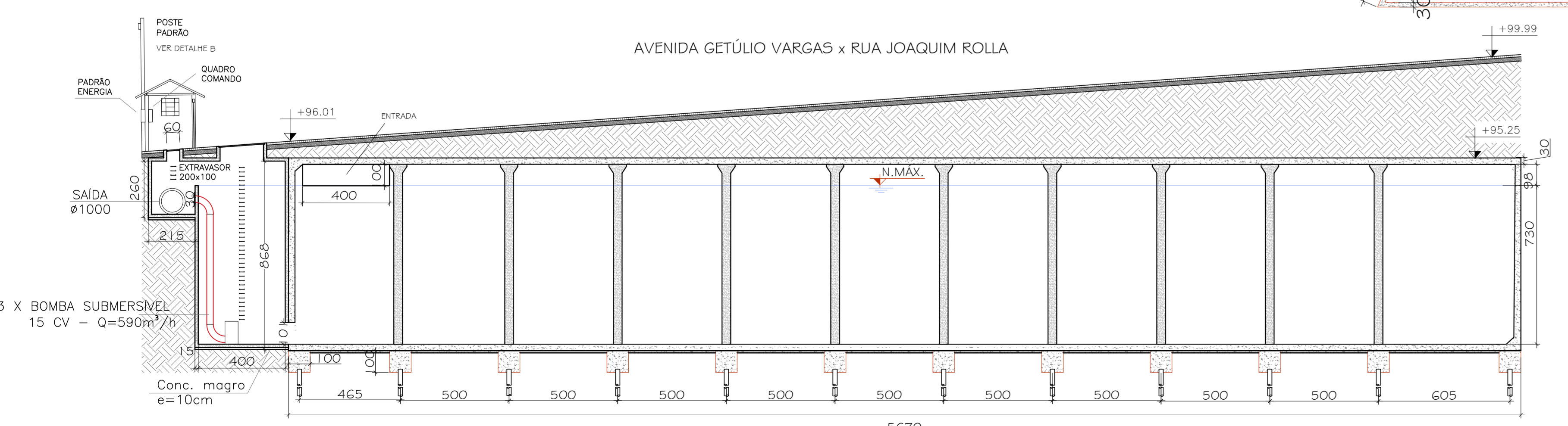
02 CORTE AA' - RAC 01 ESCALA 1/150
