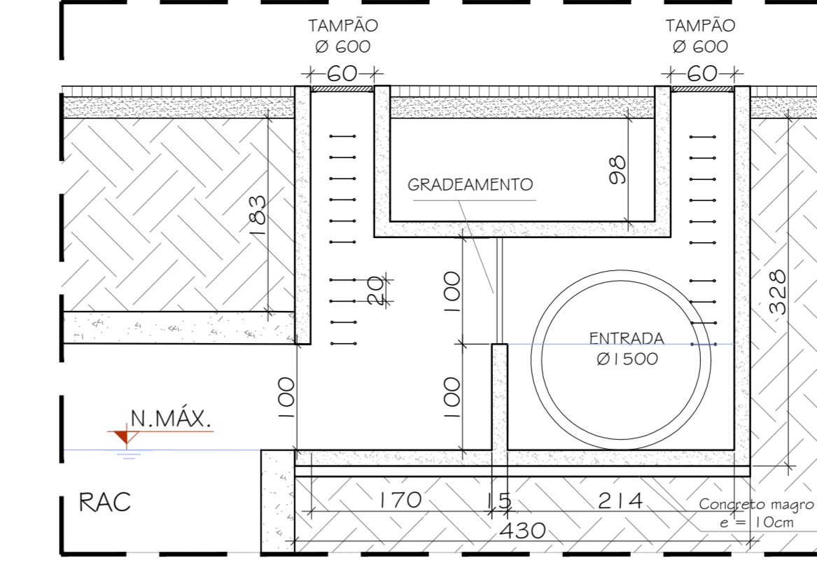
06 DETALHE A - CAIXA DE ENTRADA ESCALA 1/50
