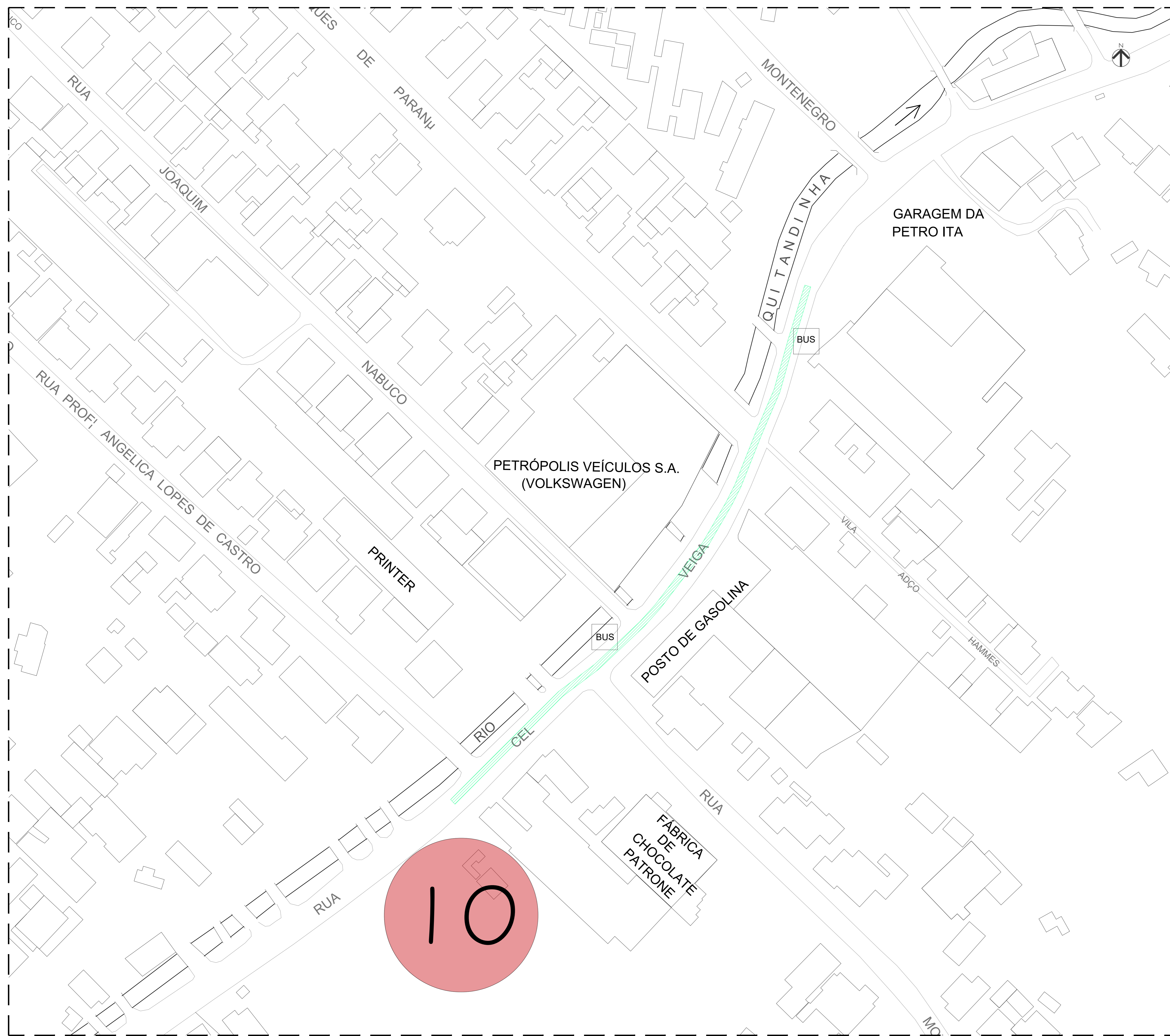
01 PLANTA DE SITUAÇÃO - GALERIA 10 ESCALA 1/500
