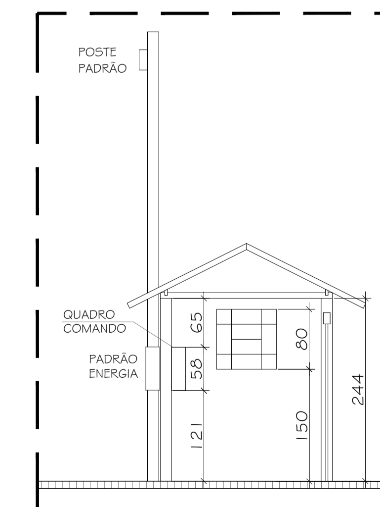
07 DETALHE C - CASA DE COMANDO ESCALA 1/50
