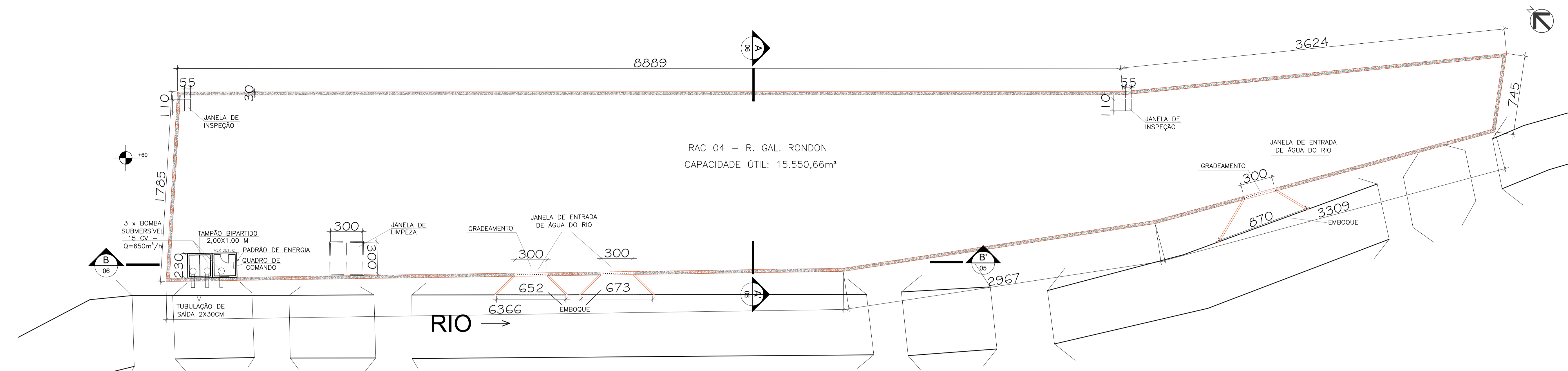
03 PLANTA BAIXA - RAC 04 ESCALA 1/200
