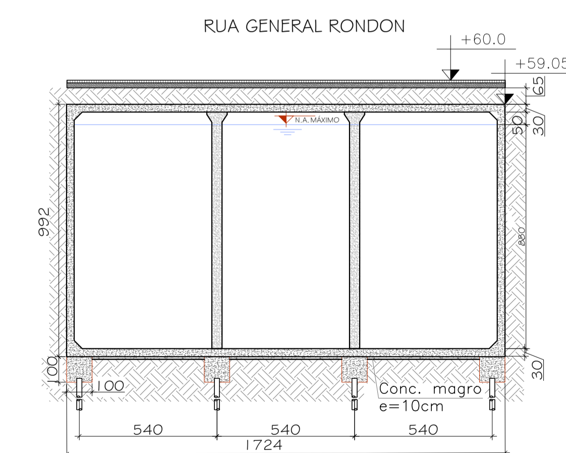
05 CORTE BB' - RAC 04 ESCALA 1/150
