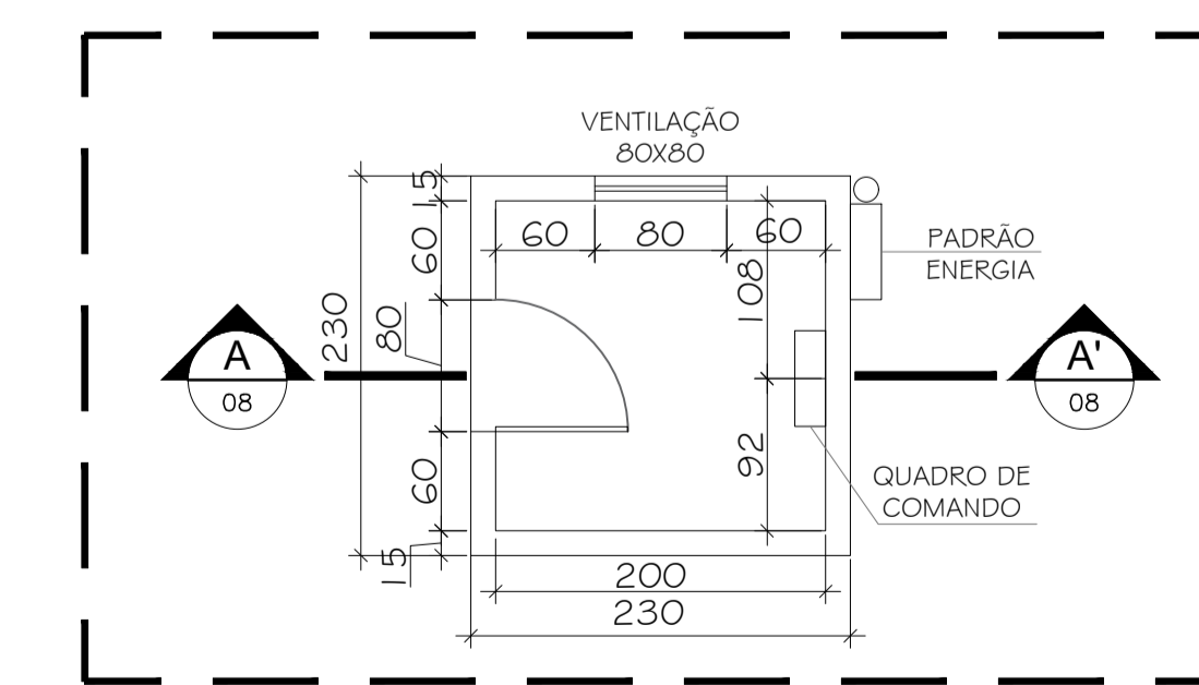
06 DETALHE C - PLANTA BAIXA CASA DE COMANDO ESCALA 1/50
