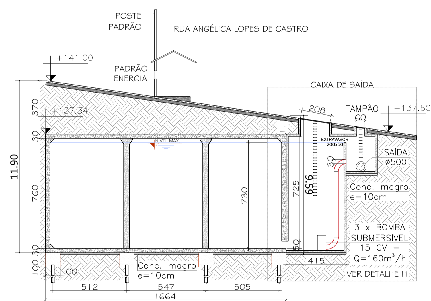
04 CORTE AA' - RAC 06 ESCALA 1/150
