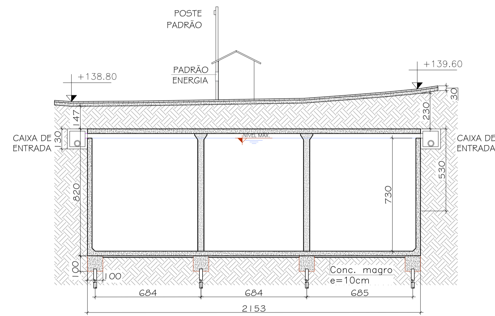
05 CORTE BB' - RAC 06 ESCALA 1/150
