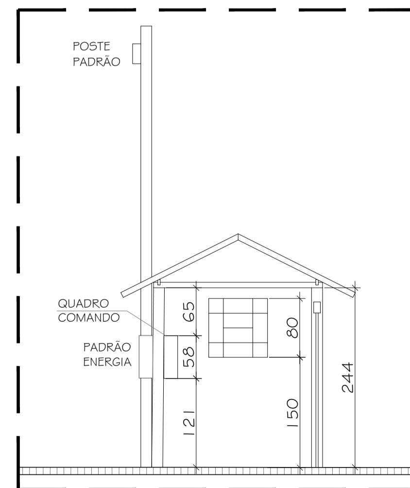
08 DETALHE C - CORTE AA' CASA DE COMANDO ESCALA 1/50
