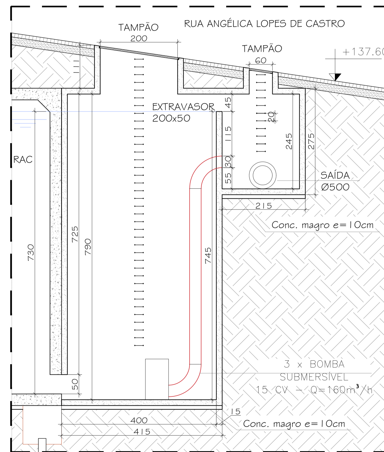
06 DETALHE H - CAIXA DE SAÍDA ESCALA 1/50
