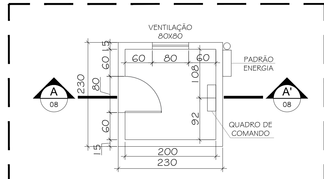
07 DETALHE C - PLANTA BAIXA CASA DE COMANDO ESCALA 1/50
