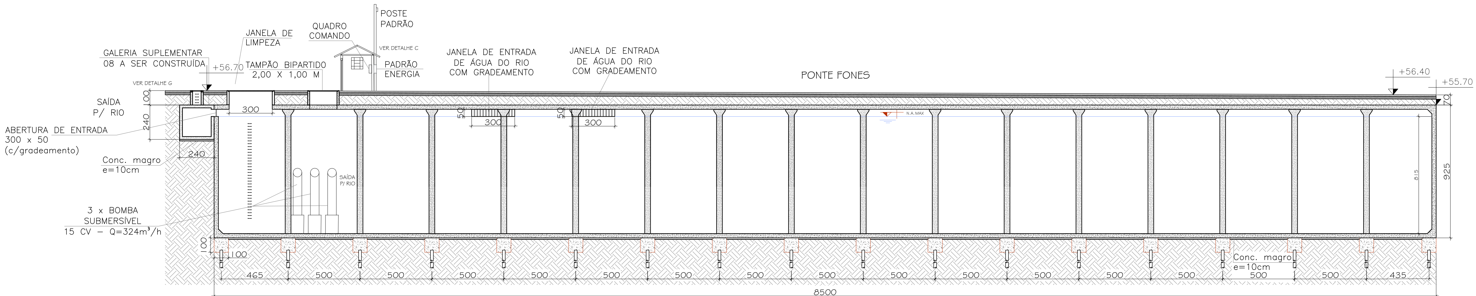
05 CORTE BB' - RAC 05 ESCALA 1/150
