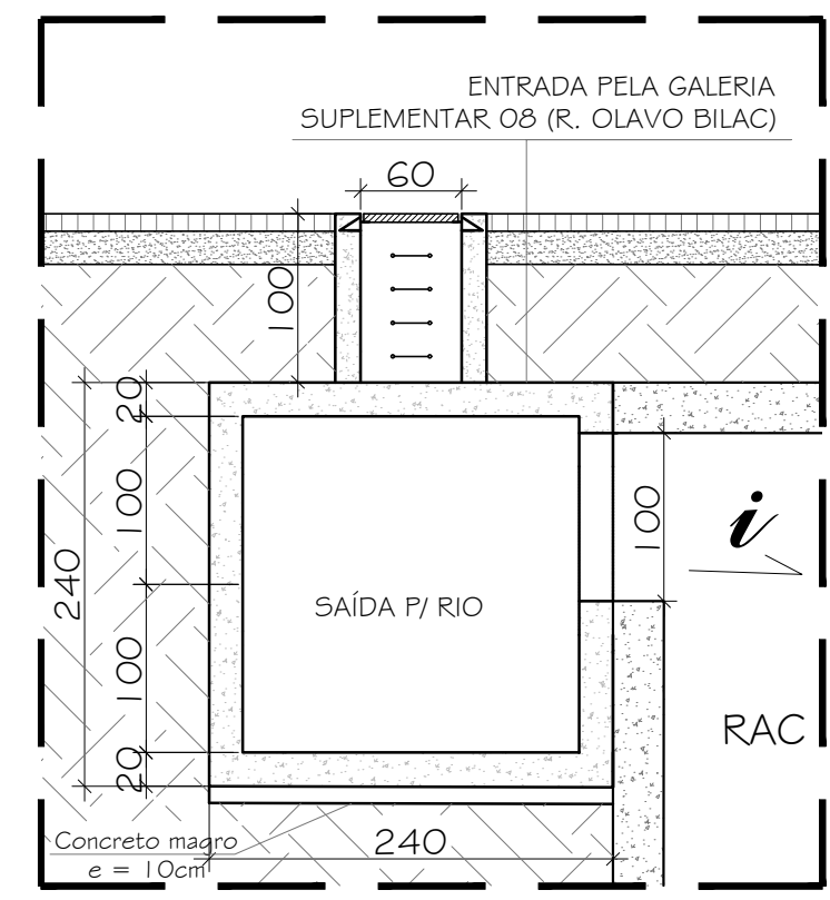
06 DETALHE G - ENTRADA RAC 05 ESCALA 1/50
