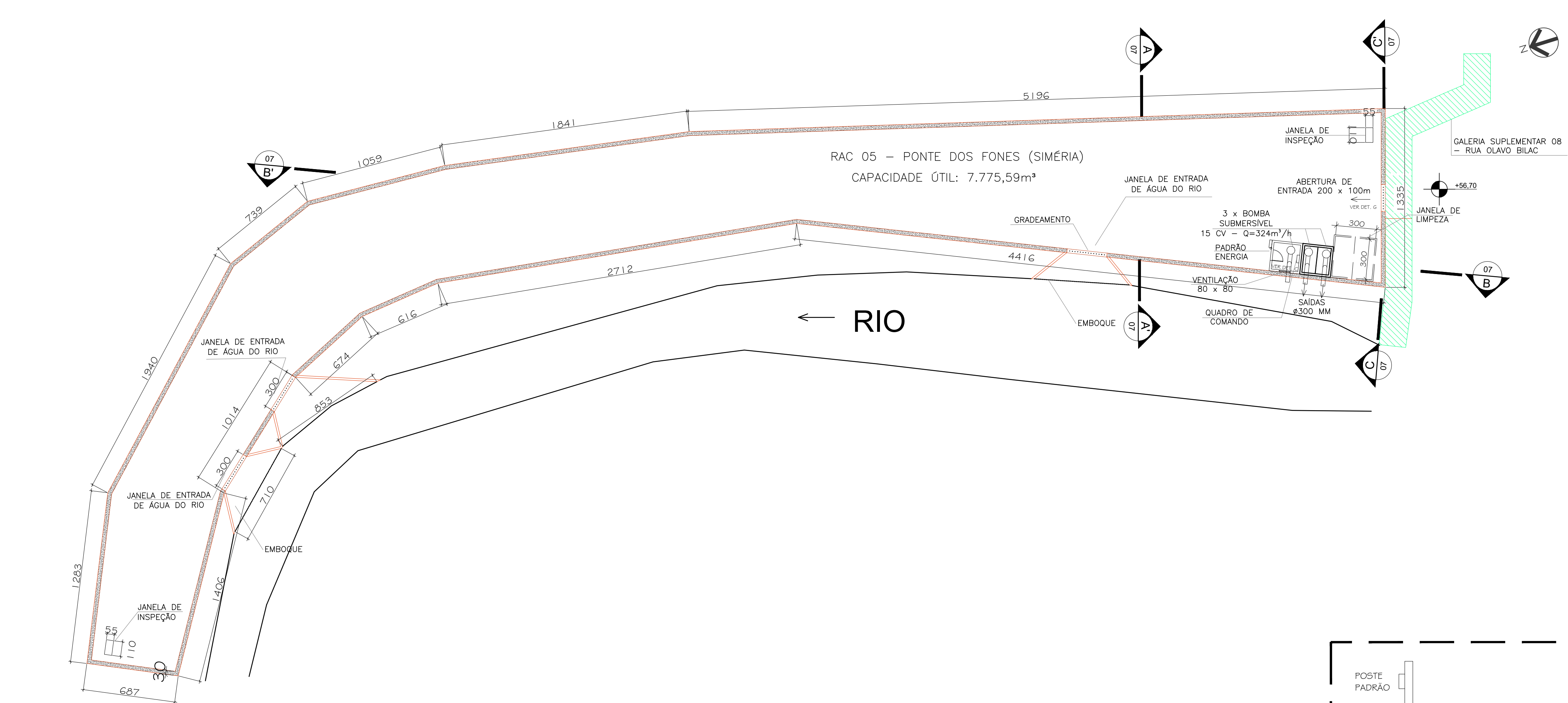
03 PLANTA BAIXA - RAC 05 ESCALA 1/200
