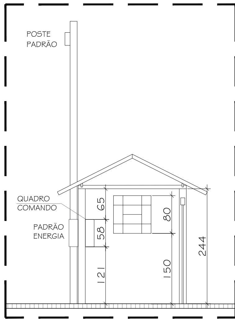
08 DETALHE C - CASA DE COMANDO ESCALA 1/50
