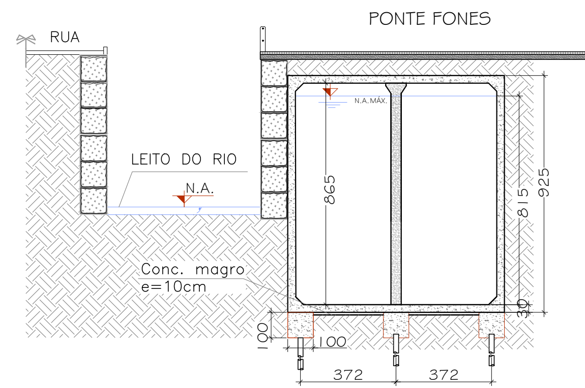
04 CORTE AA' - RAC 05 ESCALA 1/150
