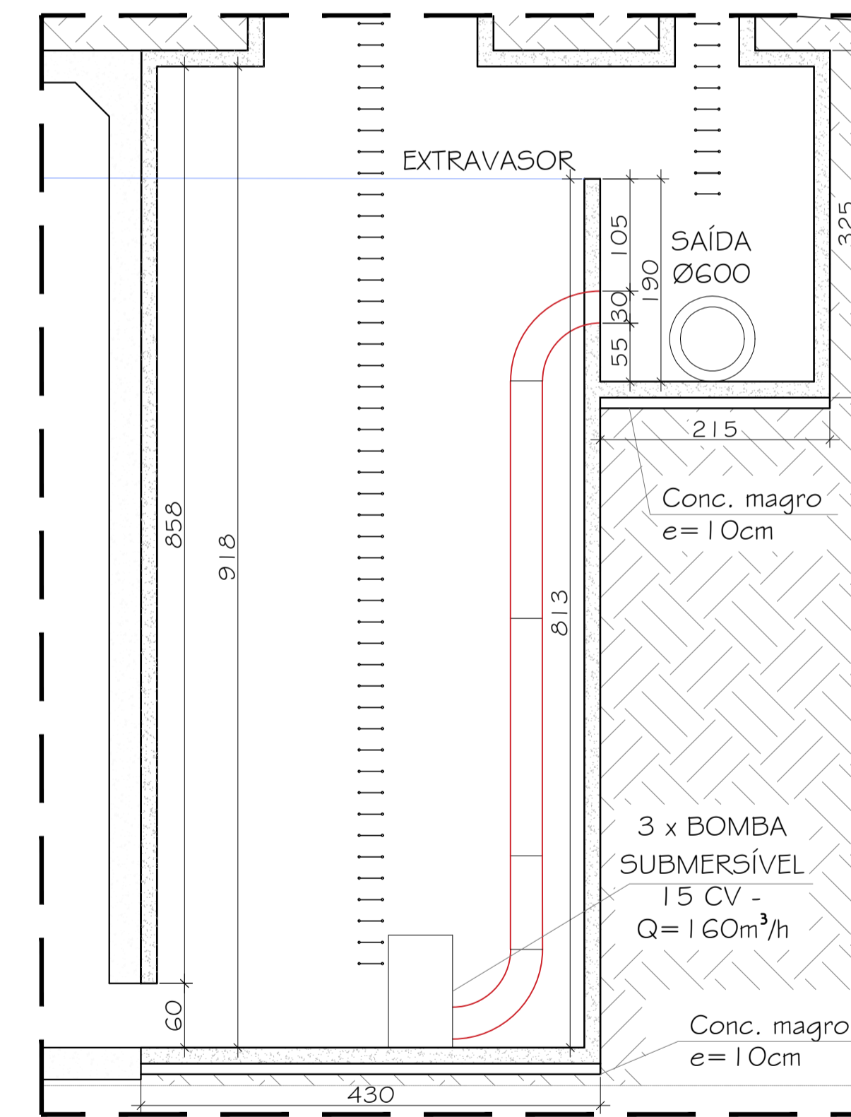
06 DETALHE L - CAIXA DE SAÍDA ESCALA 1/50
