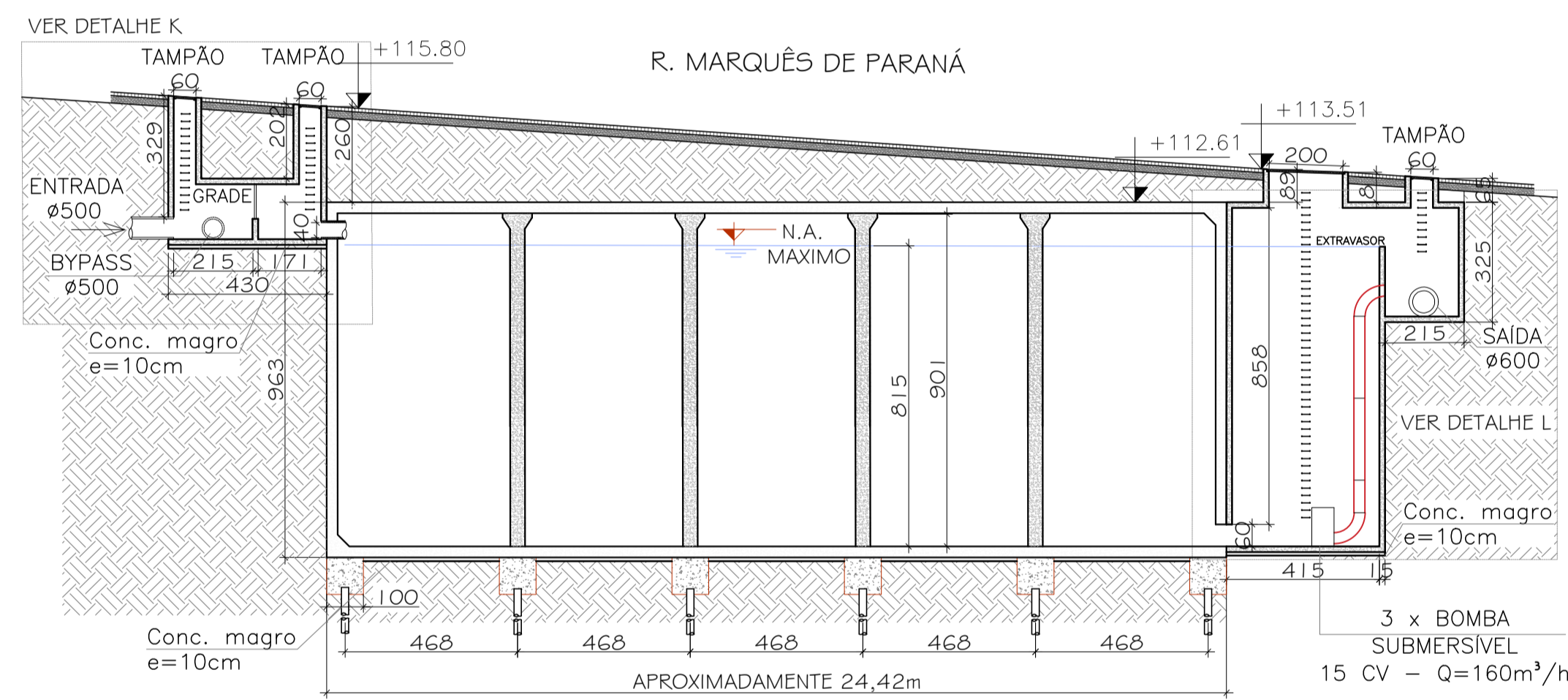
05 CORTE BB' - RAC 07 ESCALA 1/150
