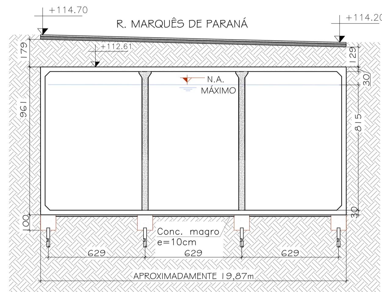
04 CORTE AA' - RAC 07 ESCALA 1/150
