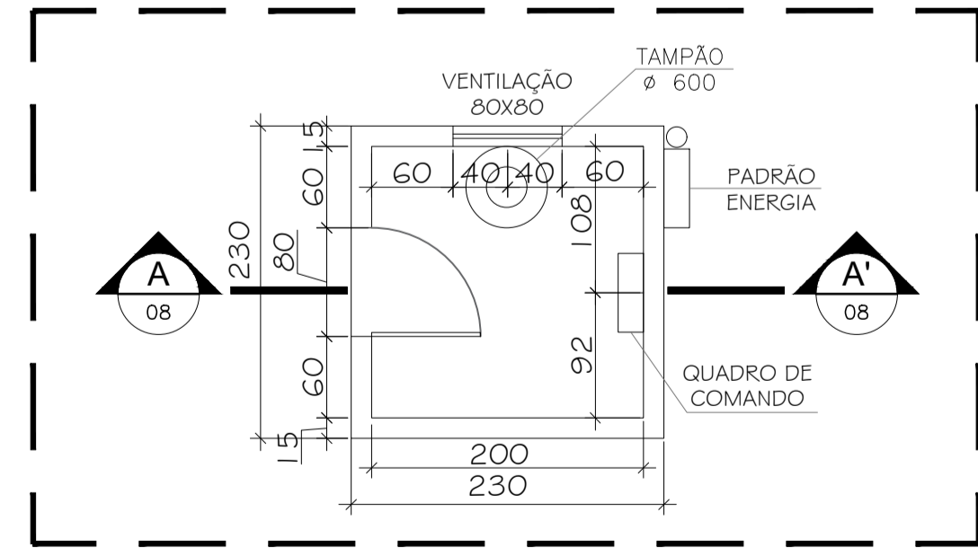
08 DETALHE D - PLANTA BAIXA CASA DE COMANDO ESCALA 1/50
