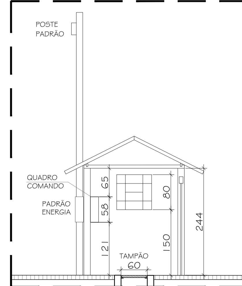
09 DETALHE D - CORTE AA' CASA DE COMANDO ESCALA 1/50
