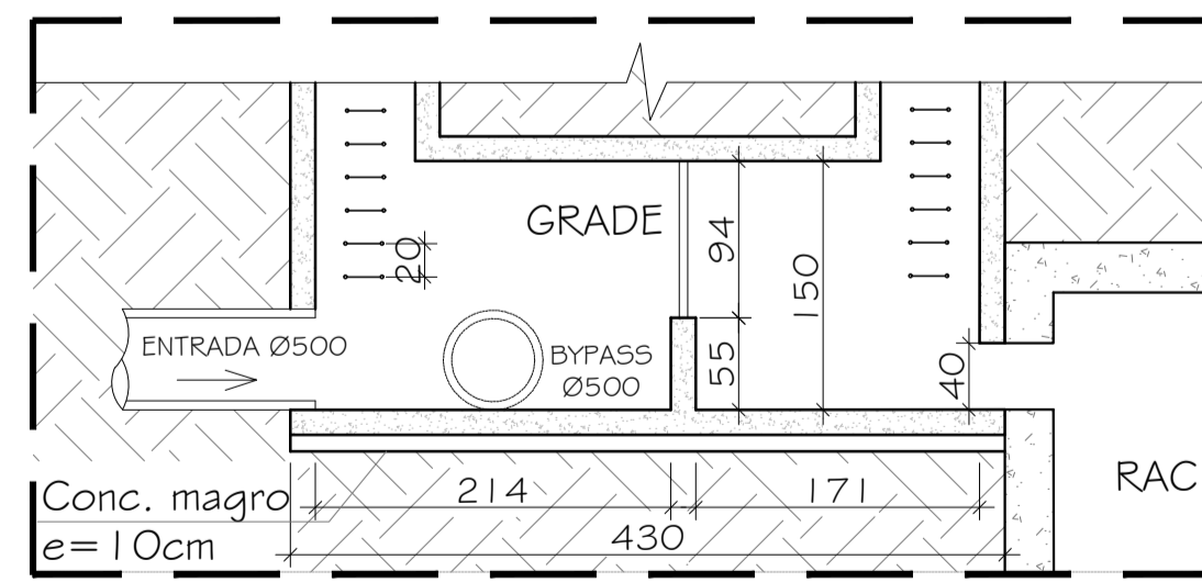
07 DETALHE K - CAIXA DE ENTRADA ESCALA 1/50
