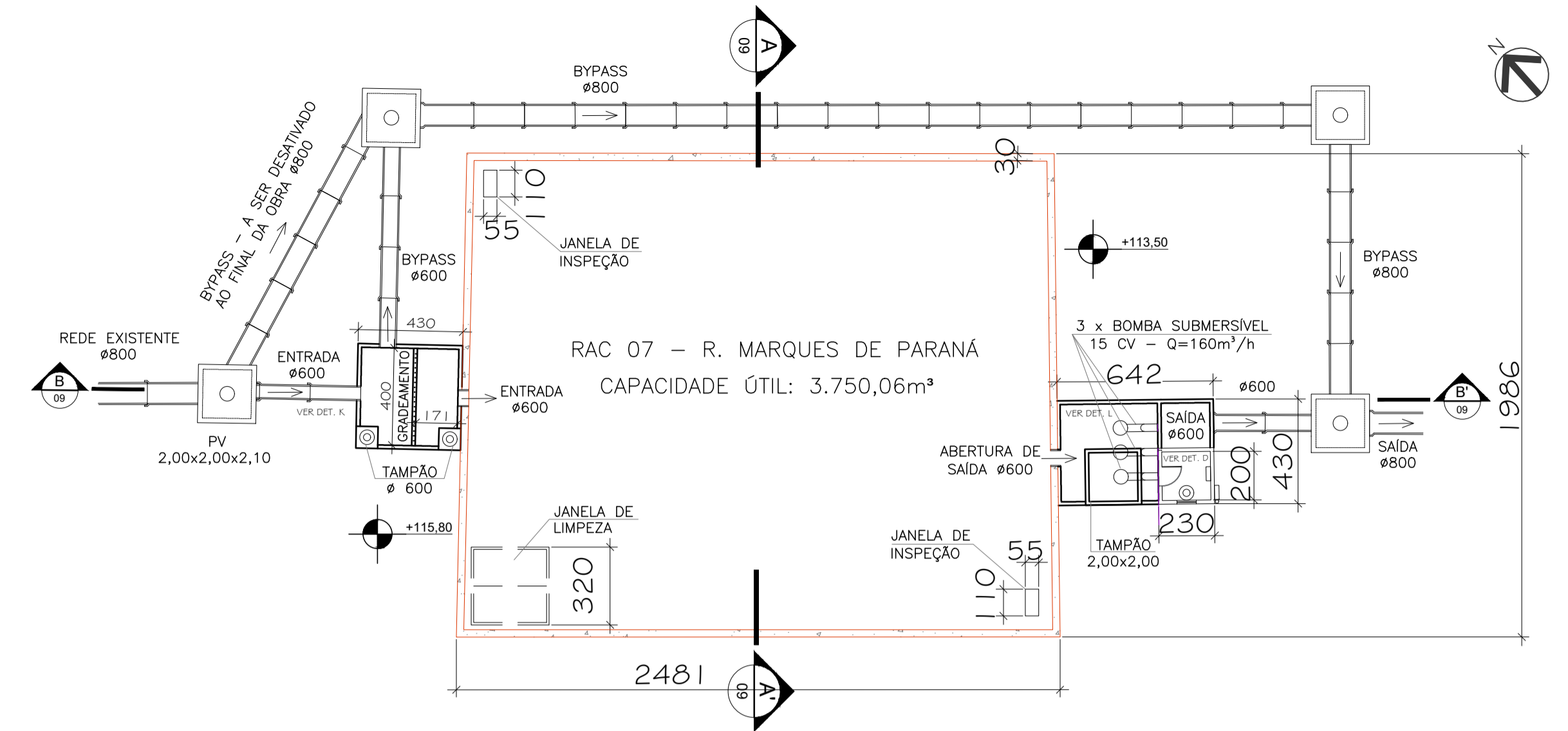
03 PLANTA BAIXA - RAC 07 ESCALA 1/200
