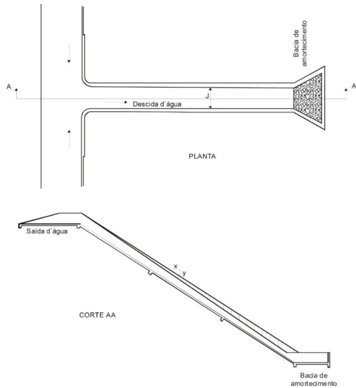
Figura – Descida d'água tipo rápido
