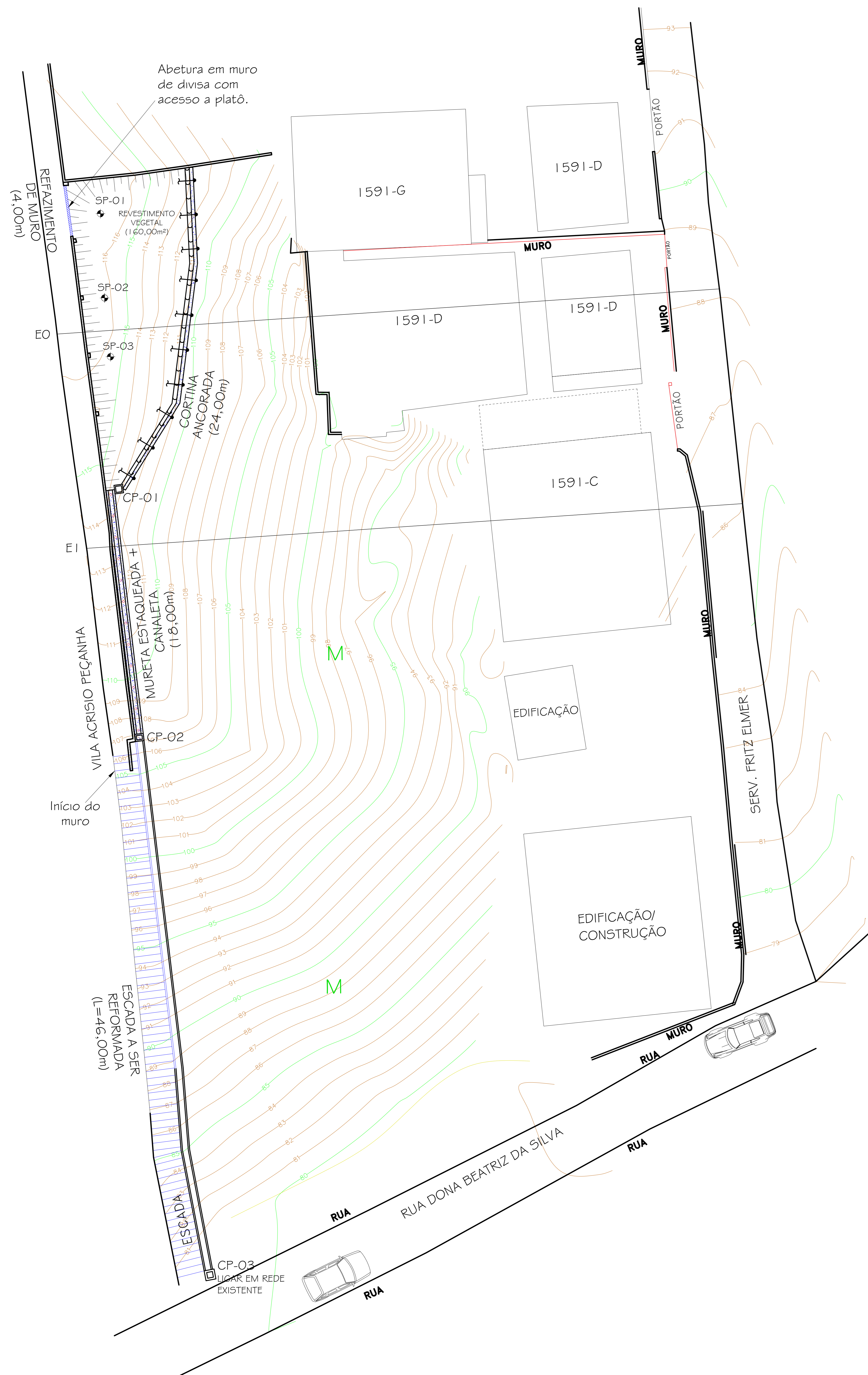
1 ARRANJO GERAL DE INTERVENÇÕES 1/125
