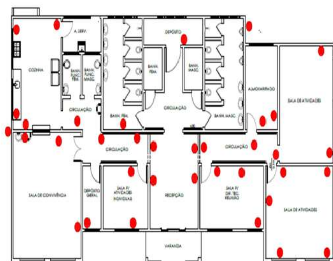
PLANTA BAIXA - INDICAÇÃO DAS FISSURAS Escala: 1/100
