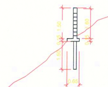
CORTE C-C
