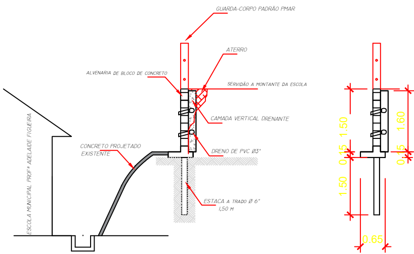
CORTE B-B
