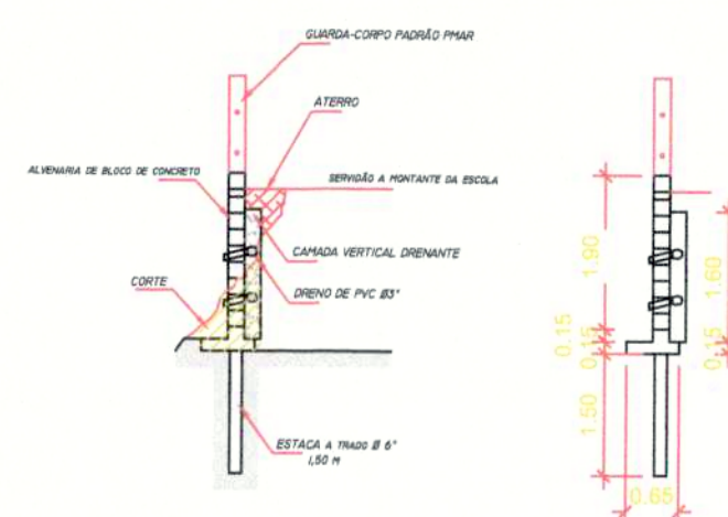
SEÇÃO TRANSVERSAL - ALVENARIA DE BLOCO DE CONCRETO ESCALA 1:100
