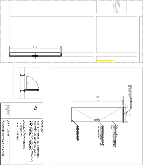
DET. 21 - ESQUADRIA - P3
