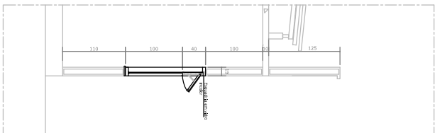
DET. 17 - ESQUADRIA - J5 ESC.:1/25
