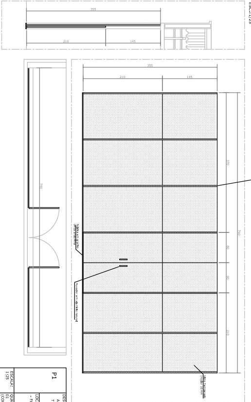
DET. 19 - ESQUADRIA - P1
