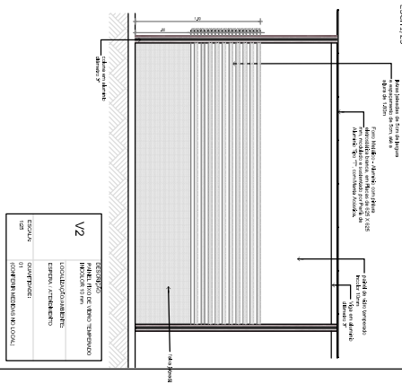
DET. 19-B - DIVISÓRIA V2
