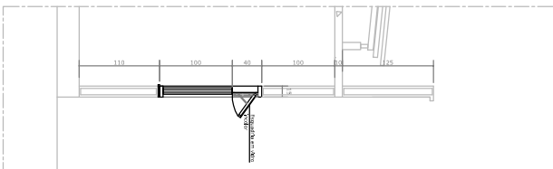
DET. 14 - ESQUADRIA - J2 ESC:1/25
