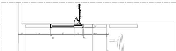
DET. 16 - ESQUADRIA - J4 ESC.:1/25
