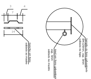
DET. 27-A - DETALHE DO MASTRO ESC.: 1/5
