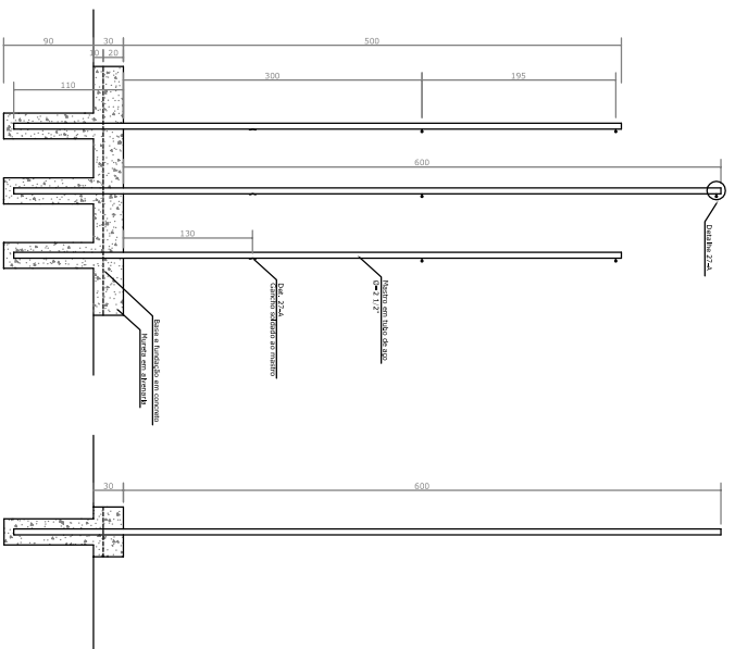
DET. 27 - MASTRO DA BANDEIRA ESC.: 1/25
