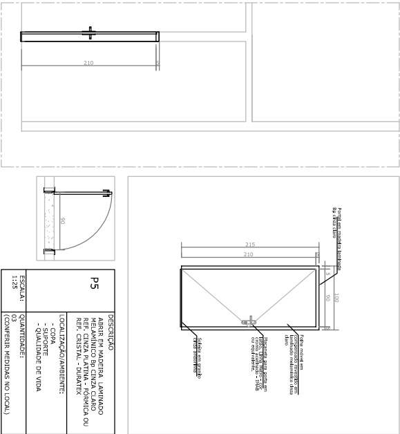
DET. 23 - ESQUADRIA - P5
