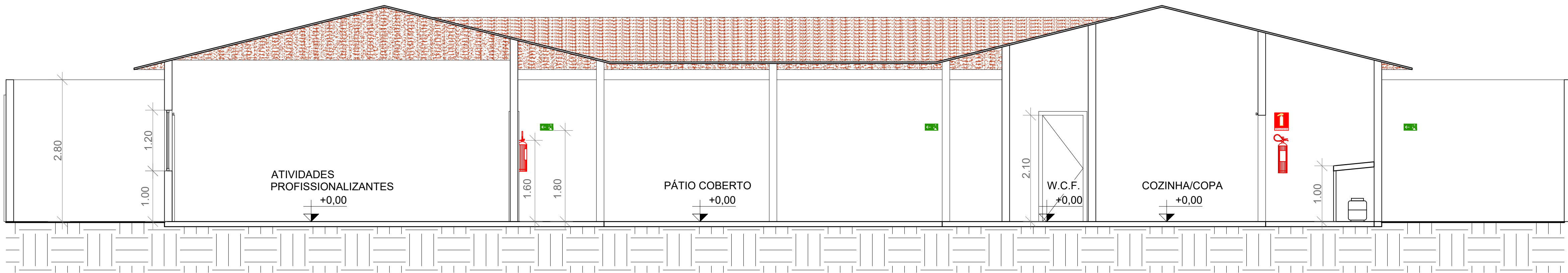
CORTE B ESCALA 1:50
