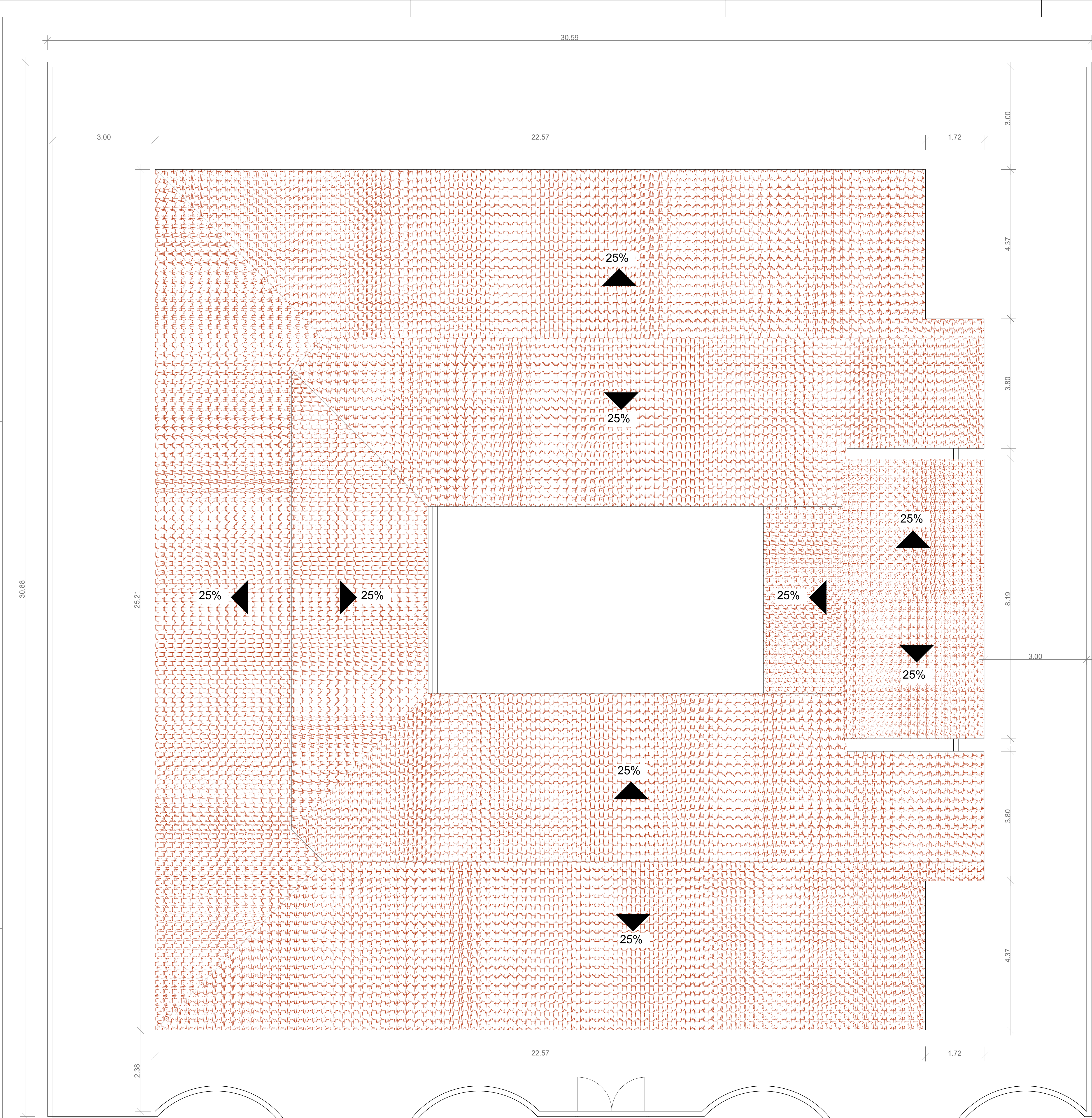
PLANTA DE IMPLANTAÇÃO/ COBERTURA ESCALA 1:50
