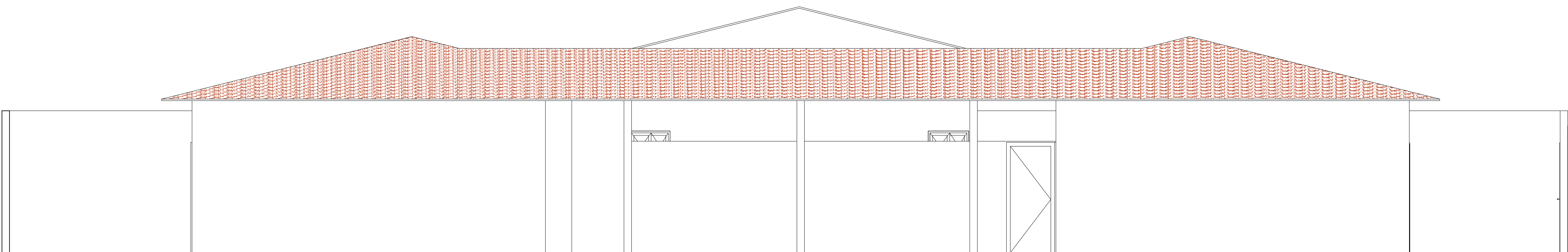
FACHADA LATERAL ESQUERDA ESCALA 1:50
