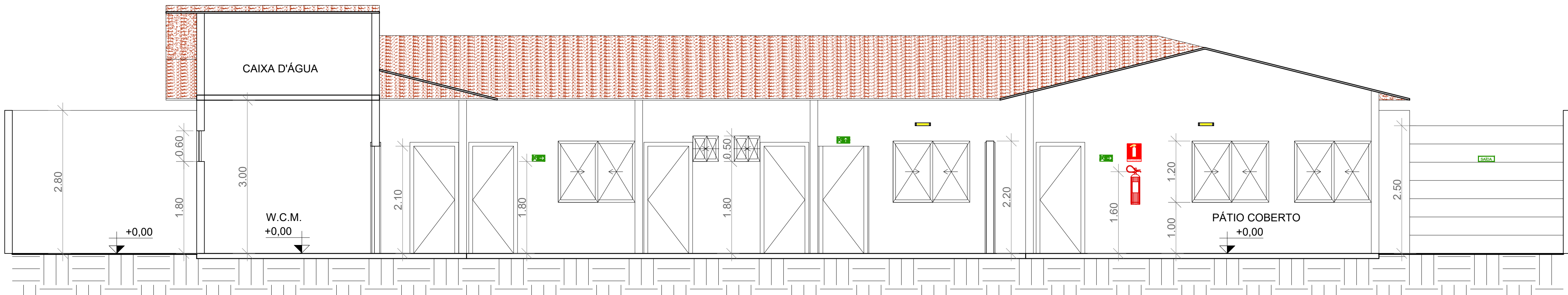
CORTE A ESCALA 1:50
