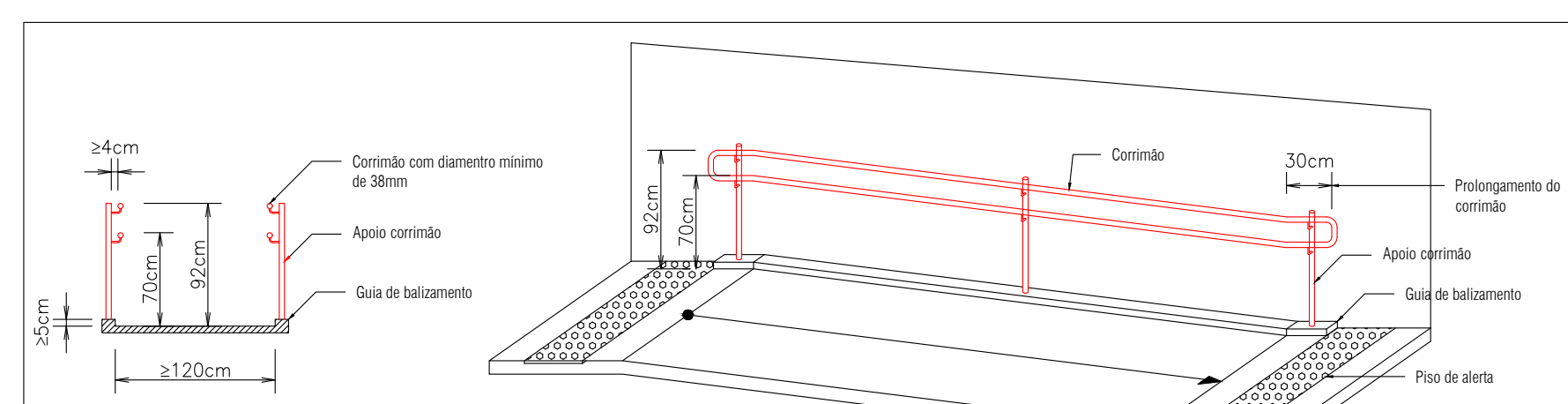
Detalhe corrimão na rampa
