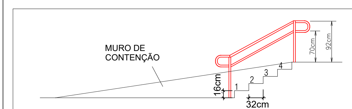
Detalhe escada 01 Sem escada
