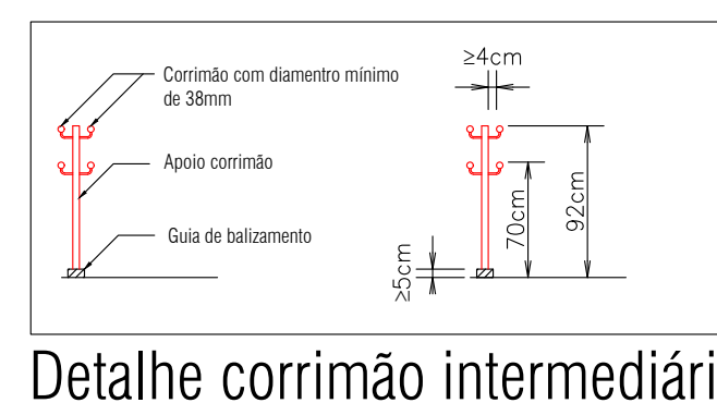
Detalhe corrimão intermediário Sem escala
