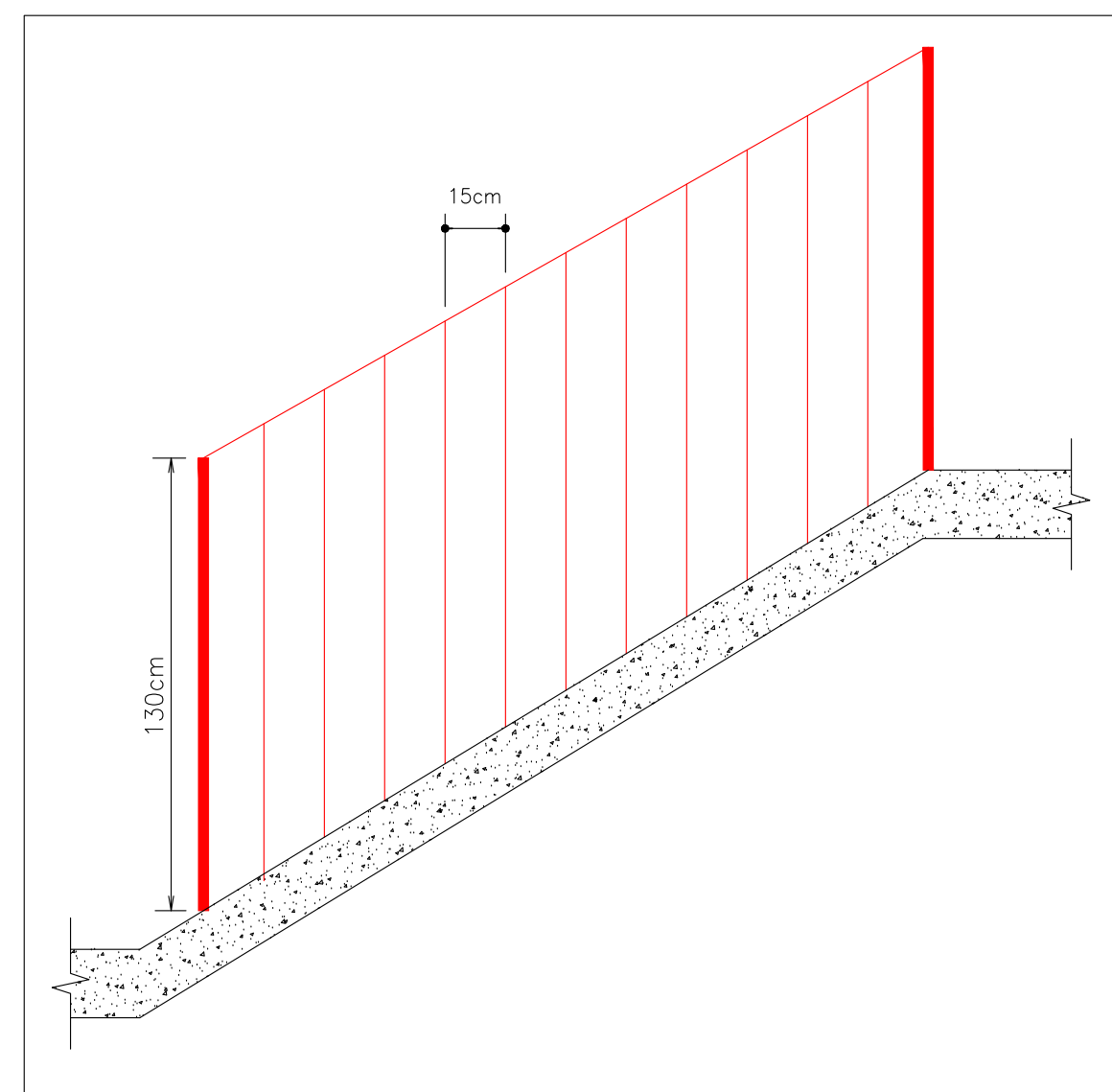
Detalhe Guarda Corpo
