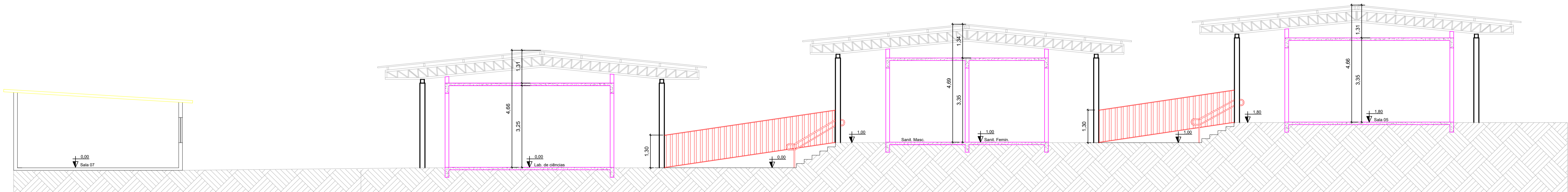
CORTE B
