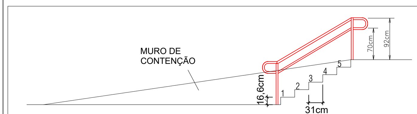
Detalhe escada 02
