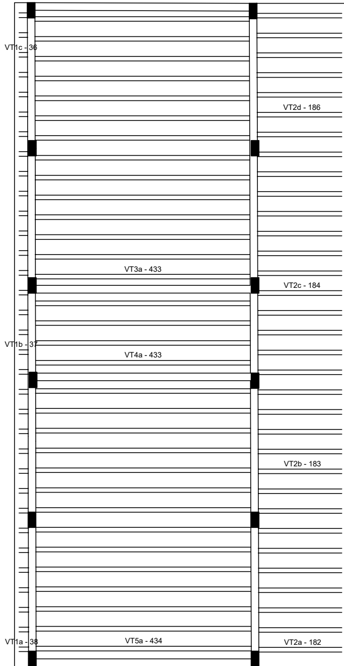
Planta de vigotas pré-moldadas
