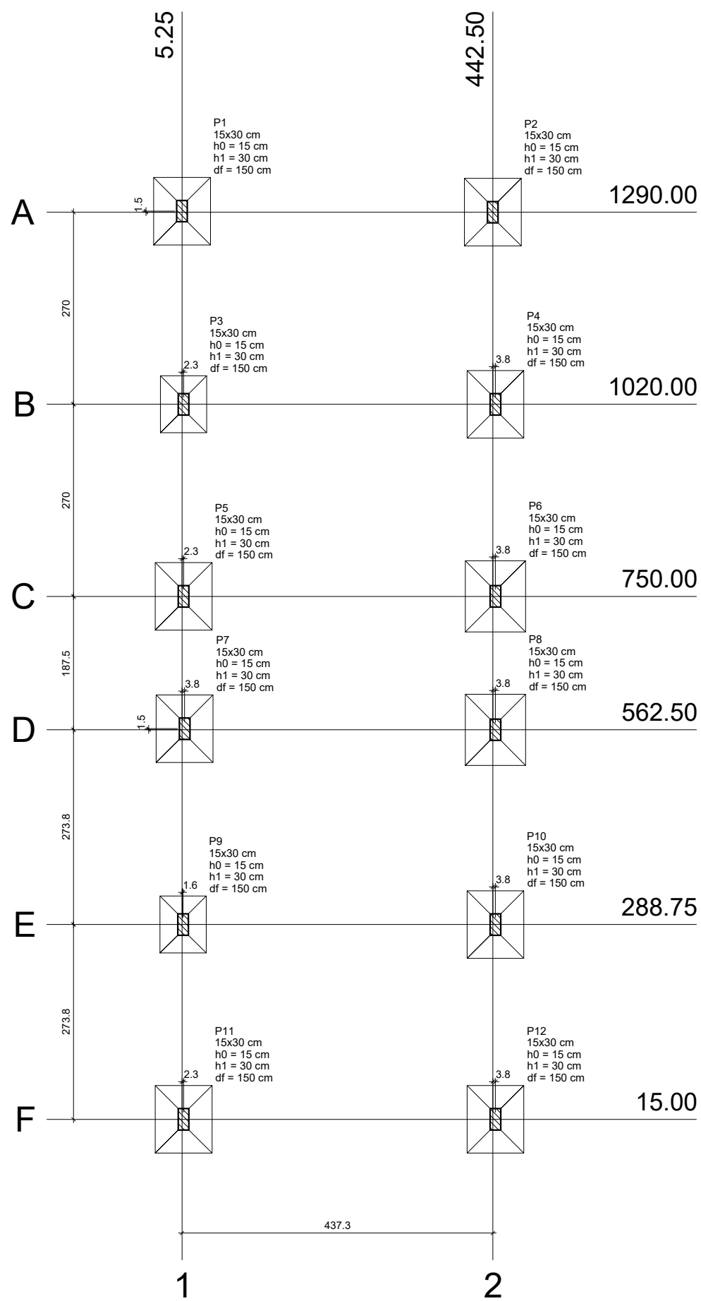
Planta de locação escala 1:50
