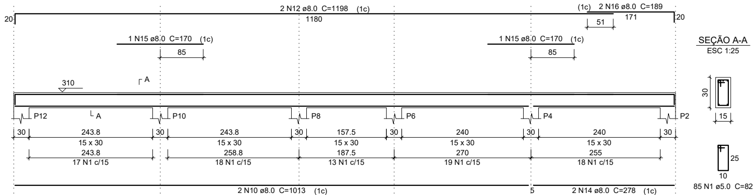
DETALHE DA ARMADURA DE SUPERIOR DE CONTINUIDADE DA LAJE E MONTAGEM DA ARMADURA DE DISTRIBUIÇÃO
