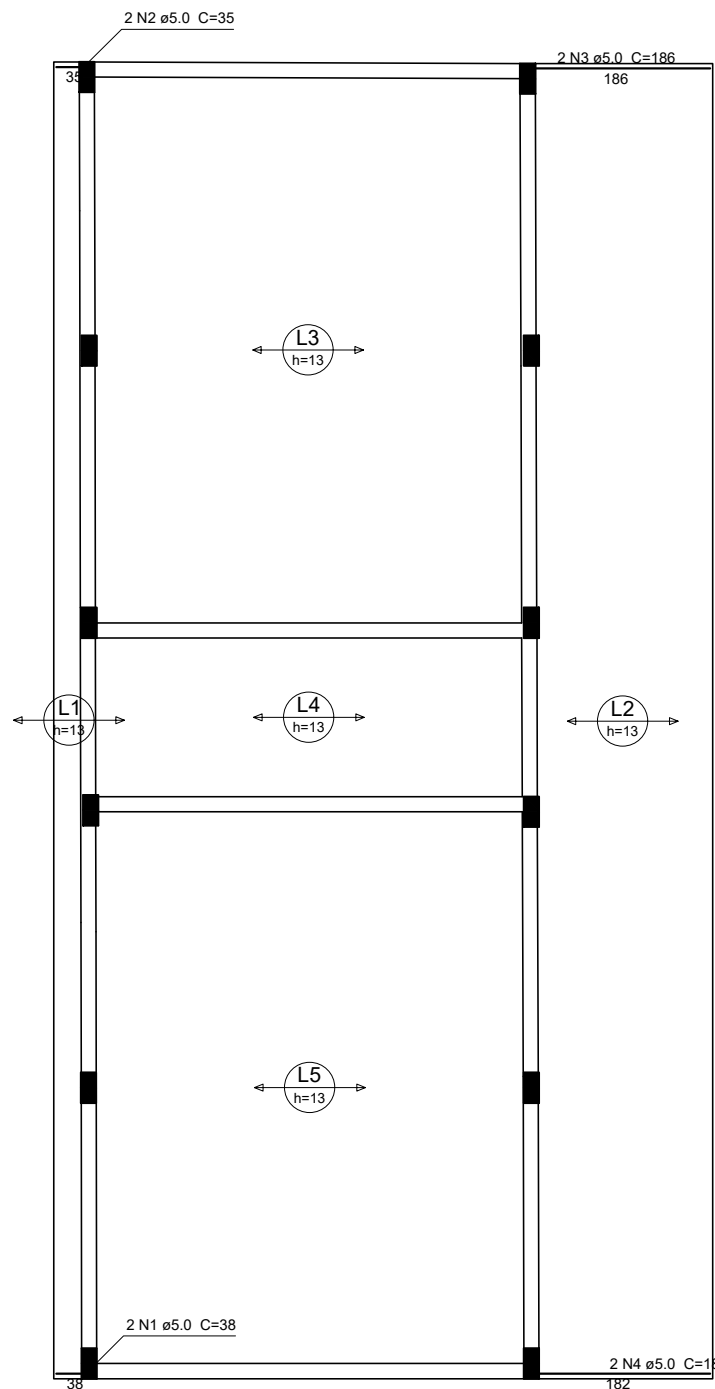
Armação positiva das lajes do pavimento Laje (Eixo X)
