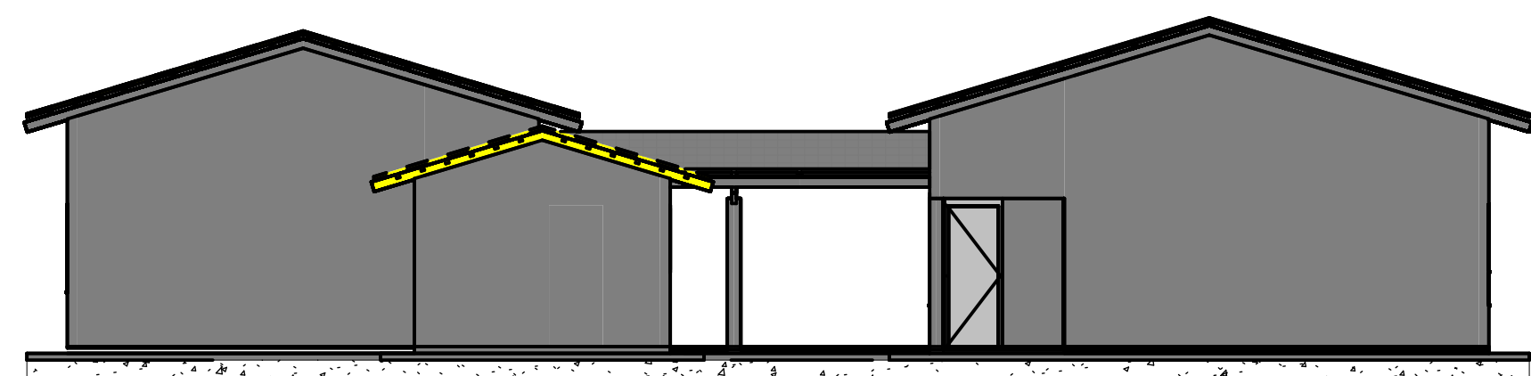
7 FACHADA LESTE DEMOLIR 1 : 100
