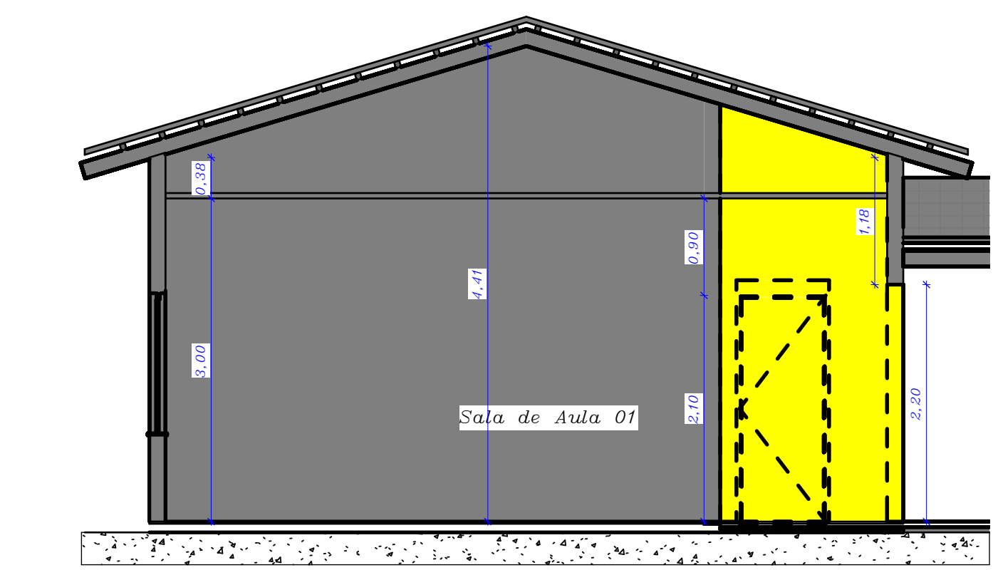
4 B-B Demolir 1 : 50
