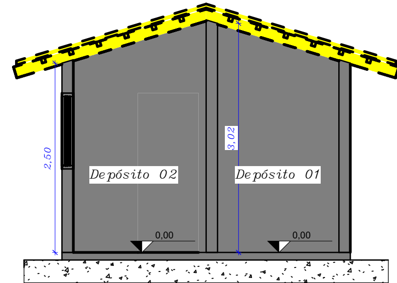
5 C-C Demolir 1 : 50
