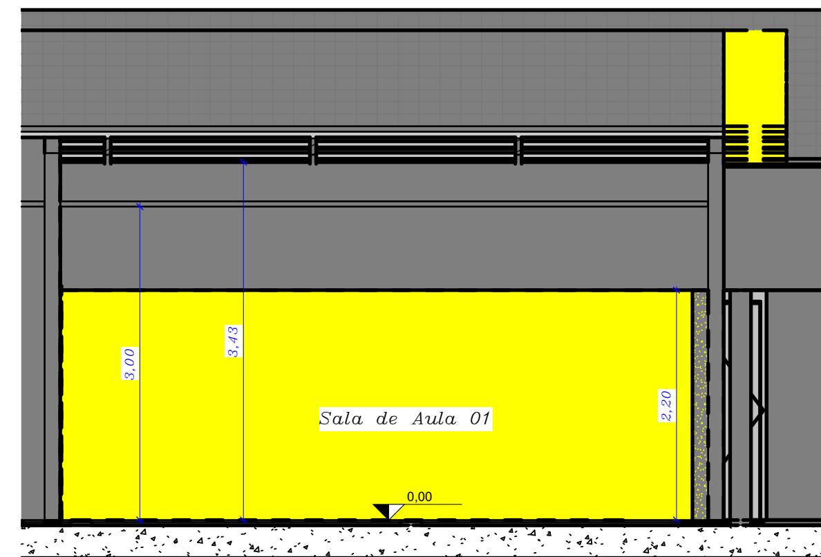
3 A-A Demolir 1 : 50
