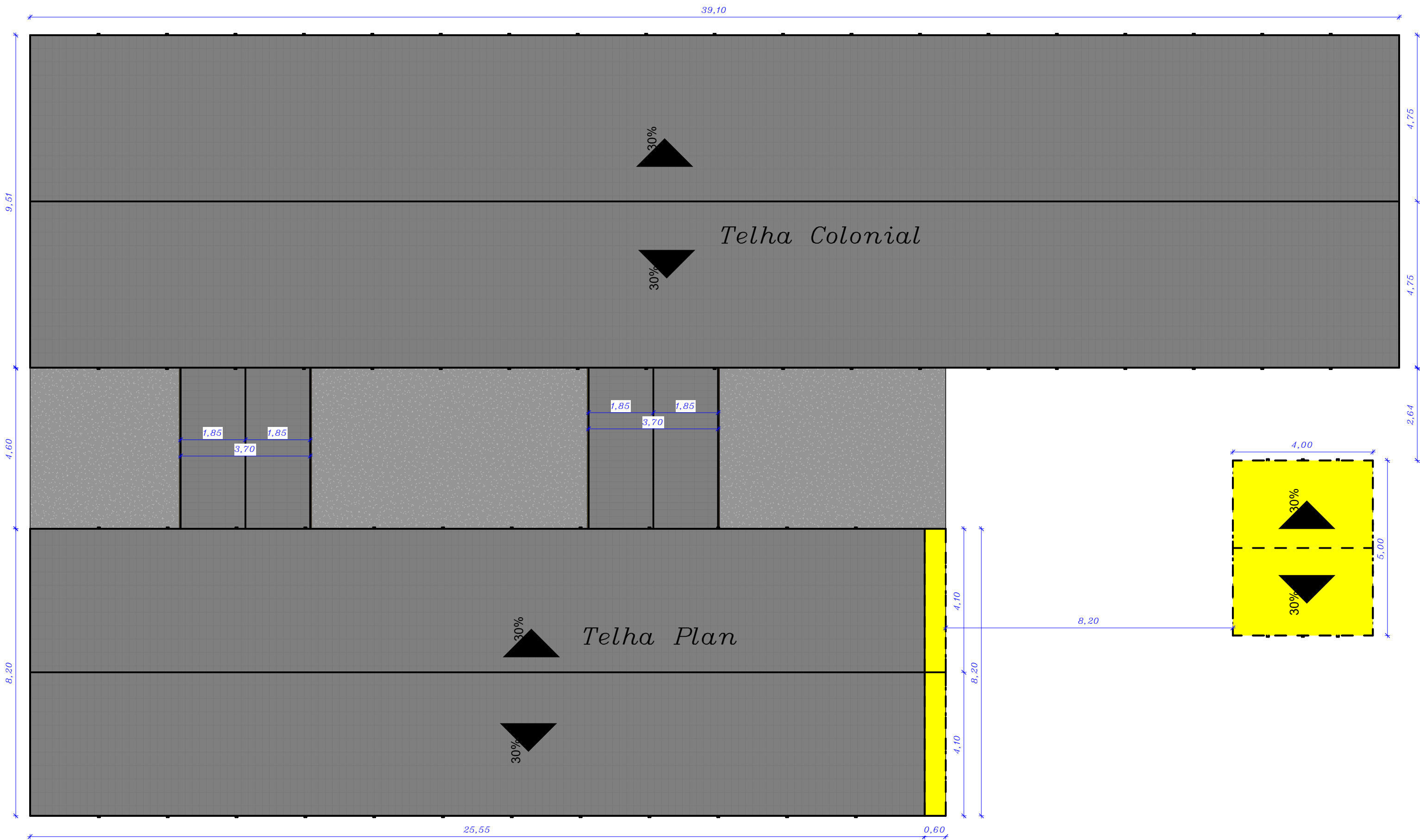
2 COBERTURA DEMOLIR 1 : 100
