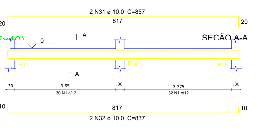
SEÇÃO A-A
