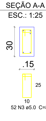
SEÇÃO A-A
