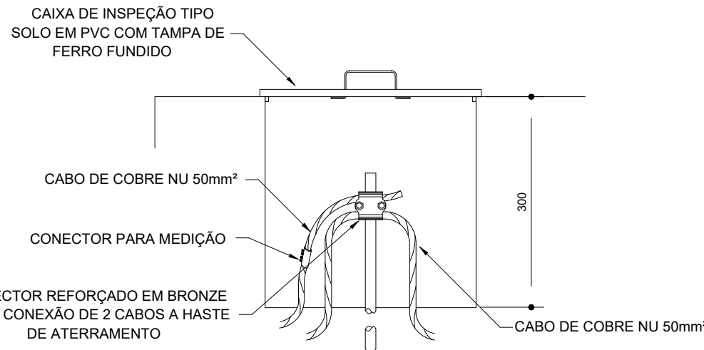
DETALHE DE INSTALAÇÃO DE CAIXA DE INSPAÇÃO TIPO SOLO COM CONECTOR DE MEDIÇÃO
