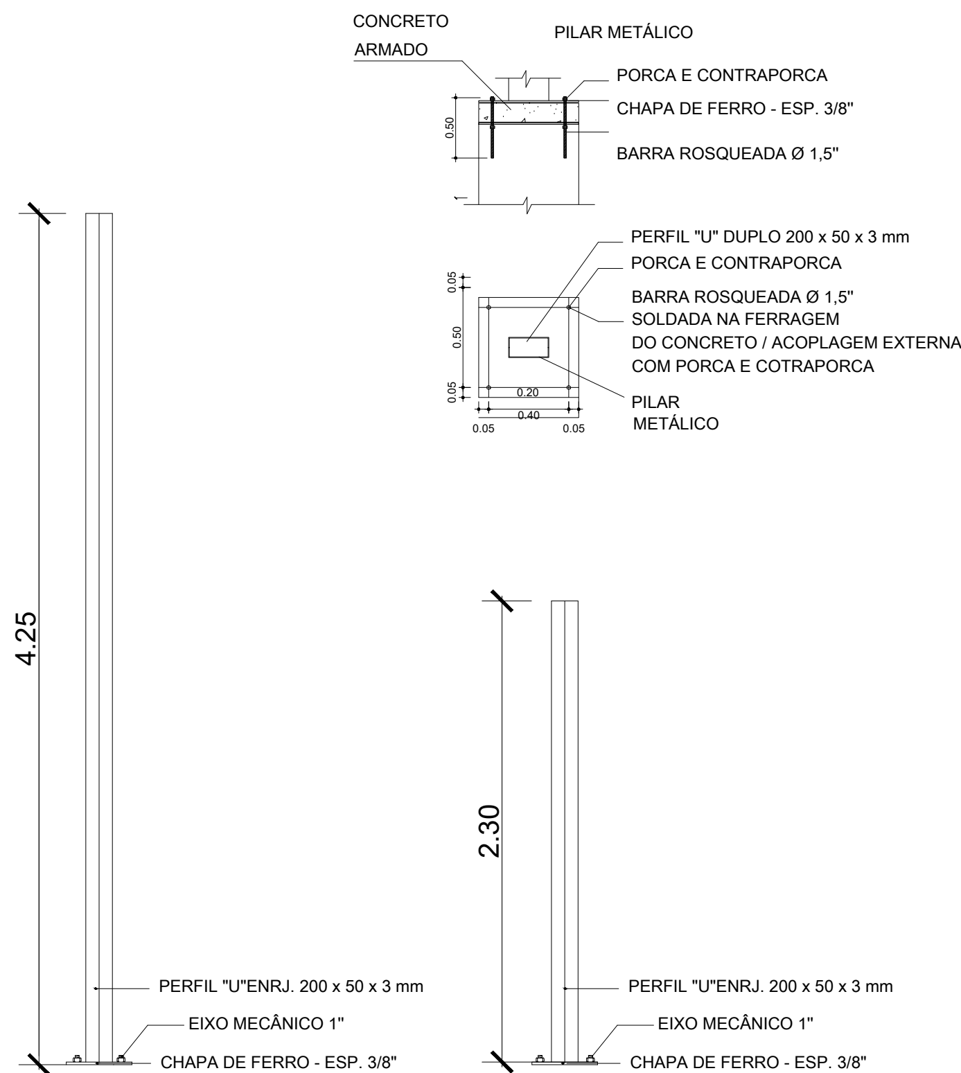
DETALHE DO PILAR METÁLICO 1 : 25
