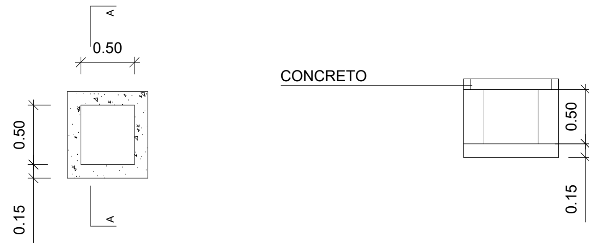
DET. CAIXA RALO ( D.I 0.50 x 0.50 x 0.50) ESC. 1/25
