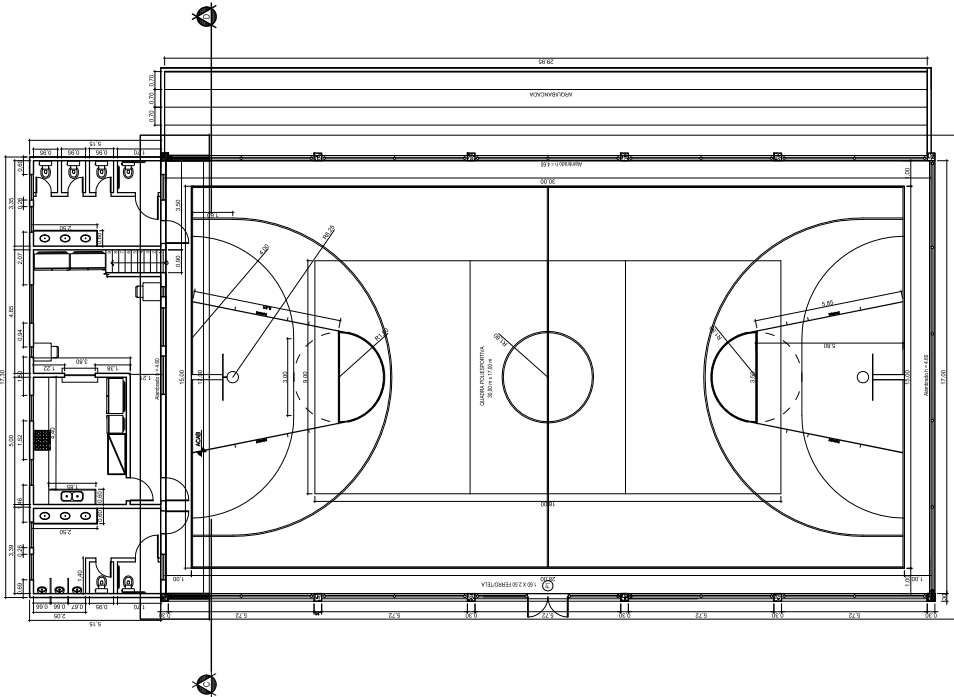
Planta Base da Quadra Poliesportiva Vargem Alta Escala: 1/50
