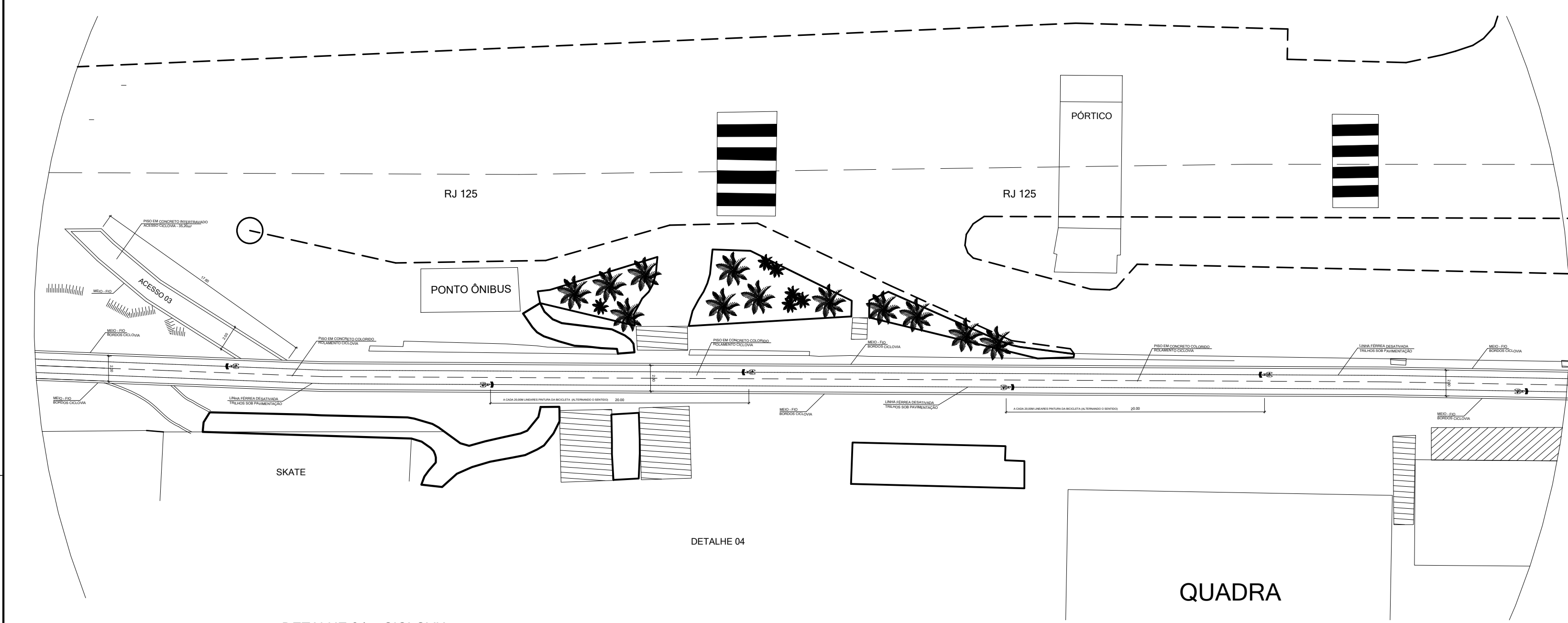
DETALHE 04 - CICLOVIA ESCALA 1:200
