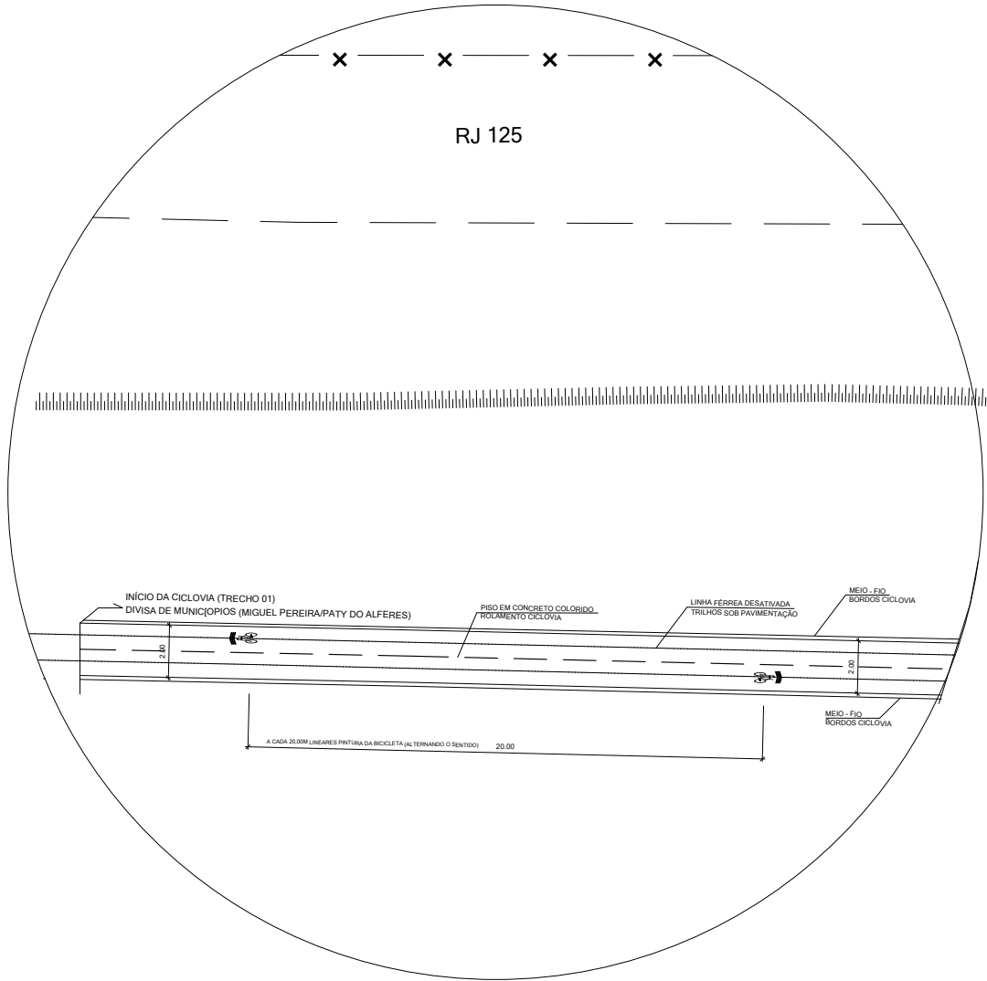
DETALHE 01 - CICLOVIA ESCALA 1:200
