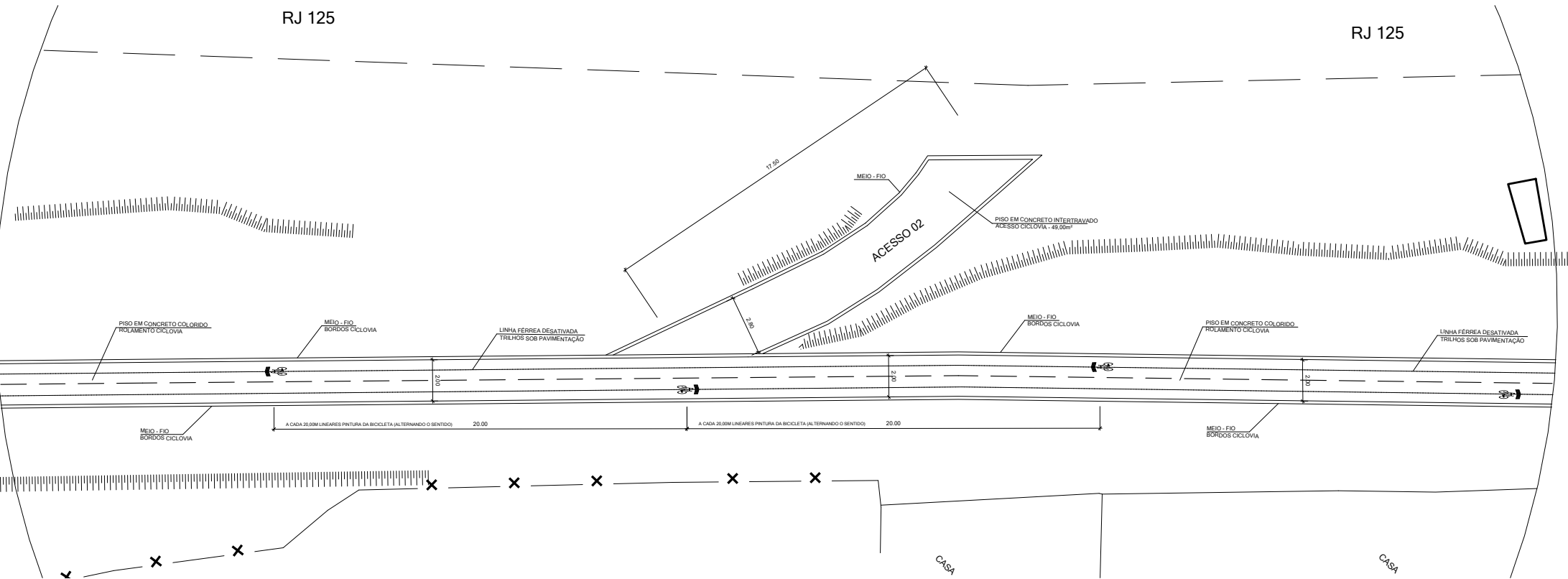
DETALHE 03 - CICLOVIA ESCALA 1:200
