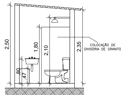
03 CORTE AA
