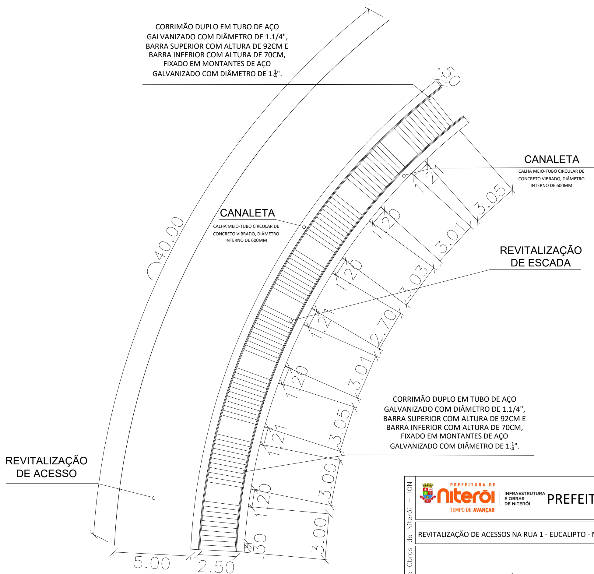
01 CROQUI ESQUEMÁTICO - EUCALIPTO - RUA 1
