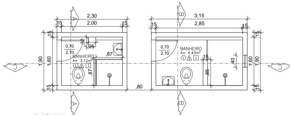
01 PLANTA BAIXA
