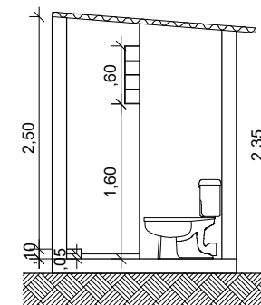
04 CORTE BB
