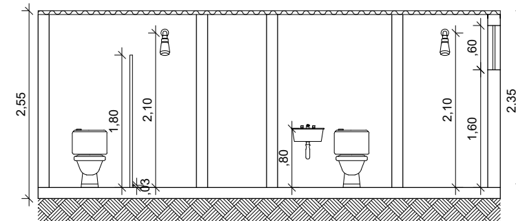
05 CORTE CC
