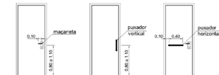
Figura 24 – Localização de maçanetas e puxadores – Exemplos
