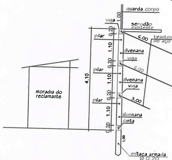
CORTE A-A SEM ESCALA
