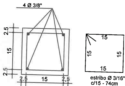
DETALHE DAS FERAGENS (cinta, vigas e pilares) sem escala
