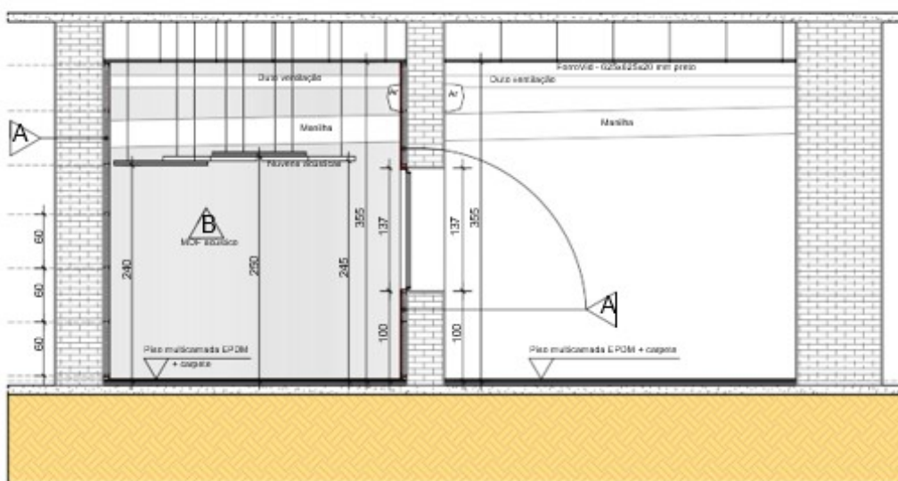
6 PAREDES ACÚSTICA CORTE ESCALA 1:75
