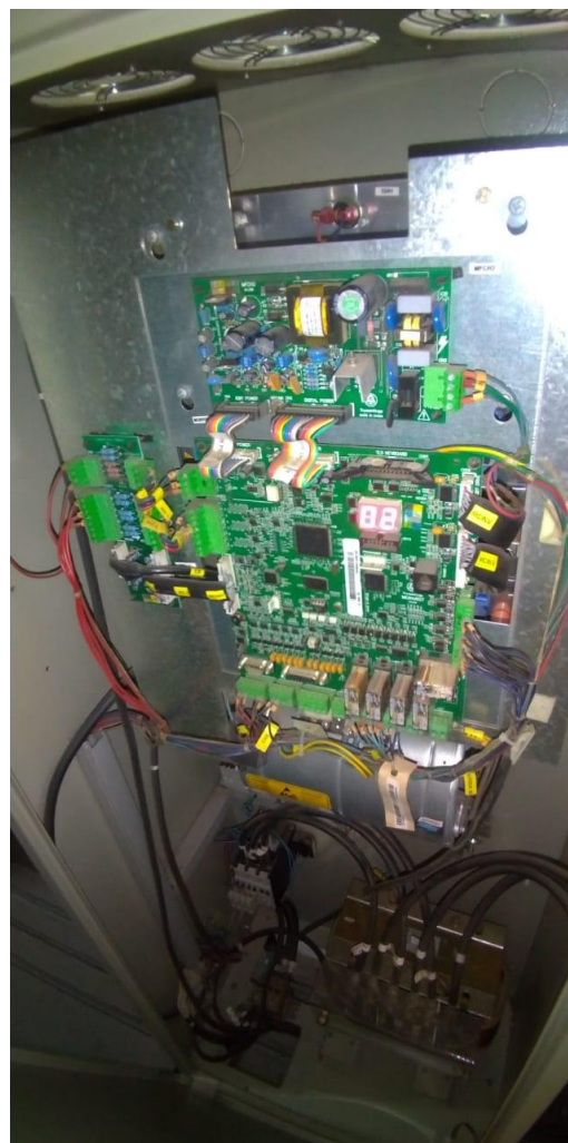
Foto 20 – Circuitos elétricos do quadro de comando
