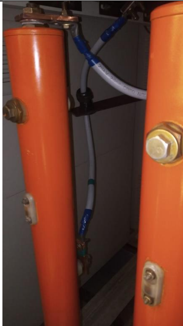
FOTO Nº 08: DETALHE DA INSTALAÇÃO DO DISJUNTOR PROVISÓRIO DE MÉDIA TENSÃO
