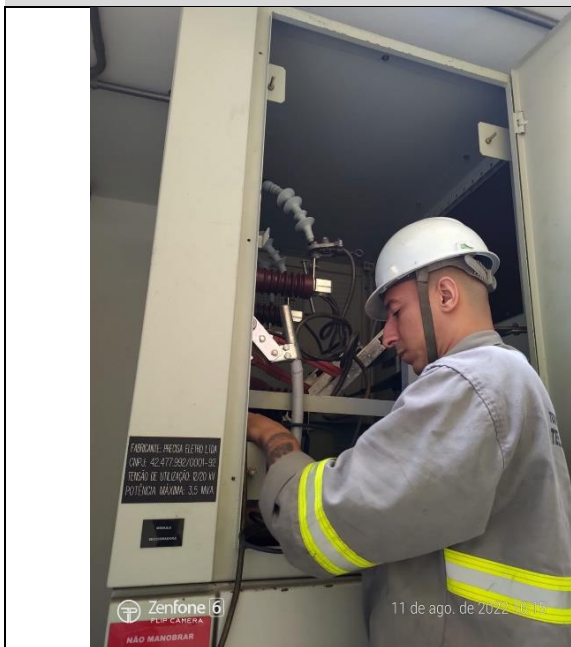
FOTO Nº 03: MANUTENÇÃO DA CHAVE SECCIONADORA
