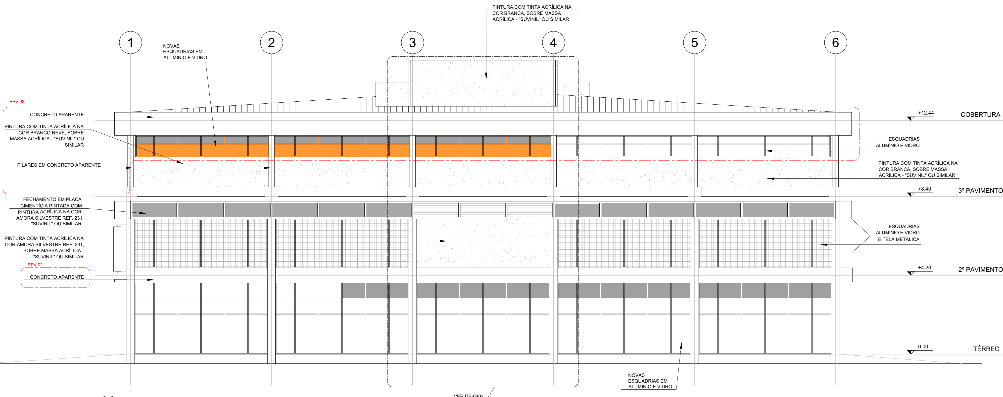
02 FACHADA SUL - ESQUERDA PE.0401/ ESCALA 1:100
