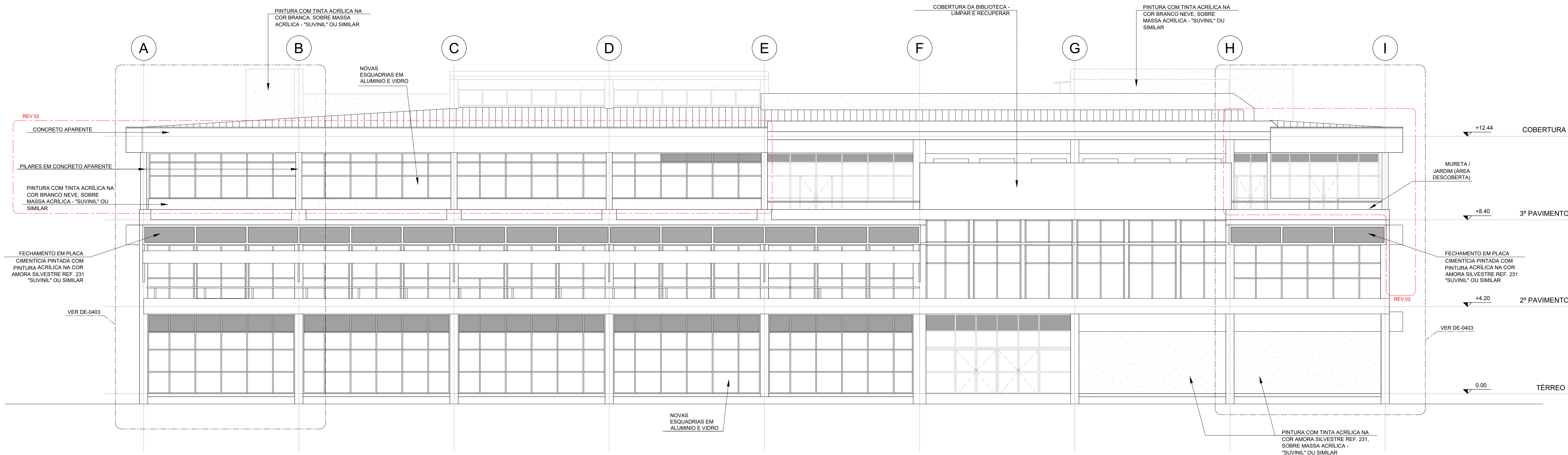
01 FACHADA LESTE - FRONTAL PE.0401/ ESCALA 1:100
