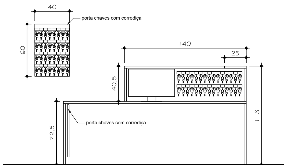
ELEVÇÃO A
