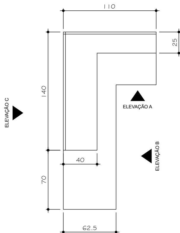
PLANTA
