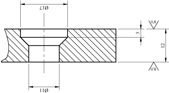
Detalhe do furo Esc. 2 : 1
