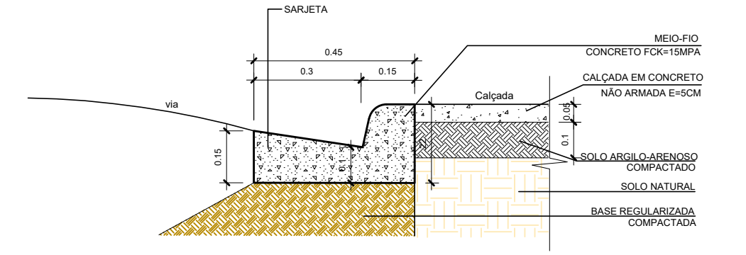
Det. Meio-fio e sarjeta Escala 1/15
