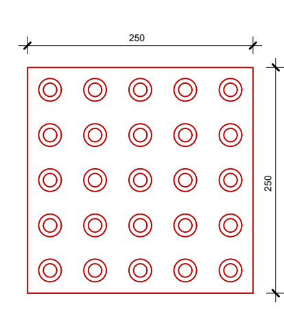
Piso Tátil de Alerta Escala 1/5
