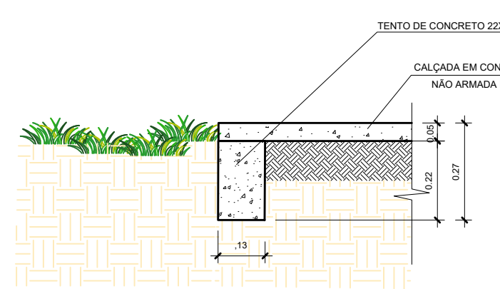
Det. Tento Calçada Escala 1/15
