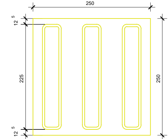
Piso Tátil Direcional Escala 1/5
