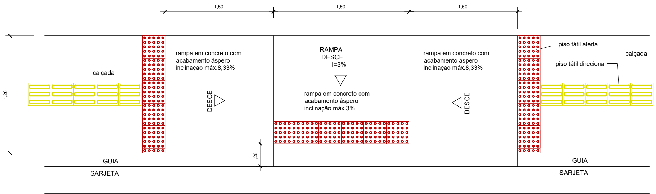
Rampa Sem Escala
