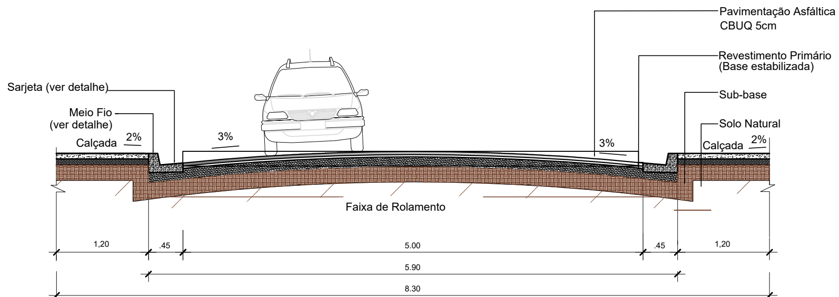
Corte da Via Escala 1/50
