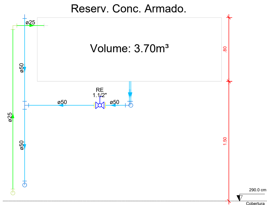
Detalhe HID-6 Escala: 1/25
