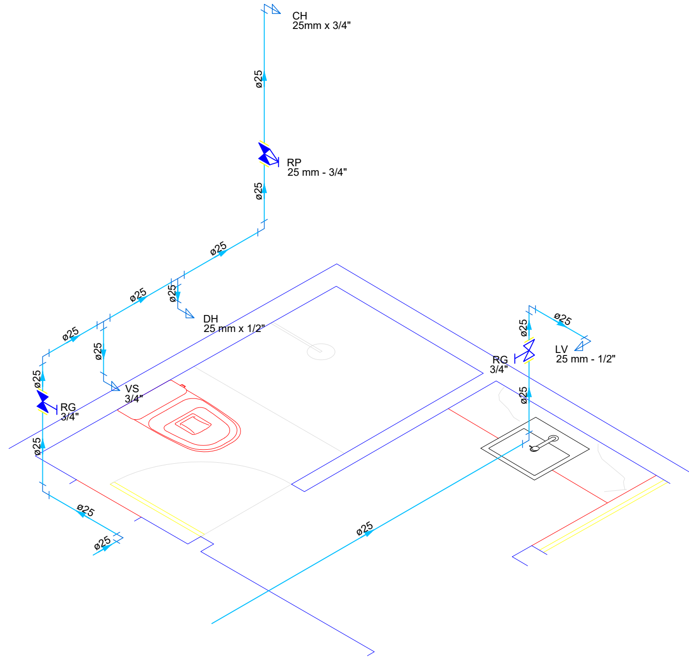
Detalhe HID-3 Escala: 1/25
