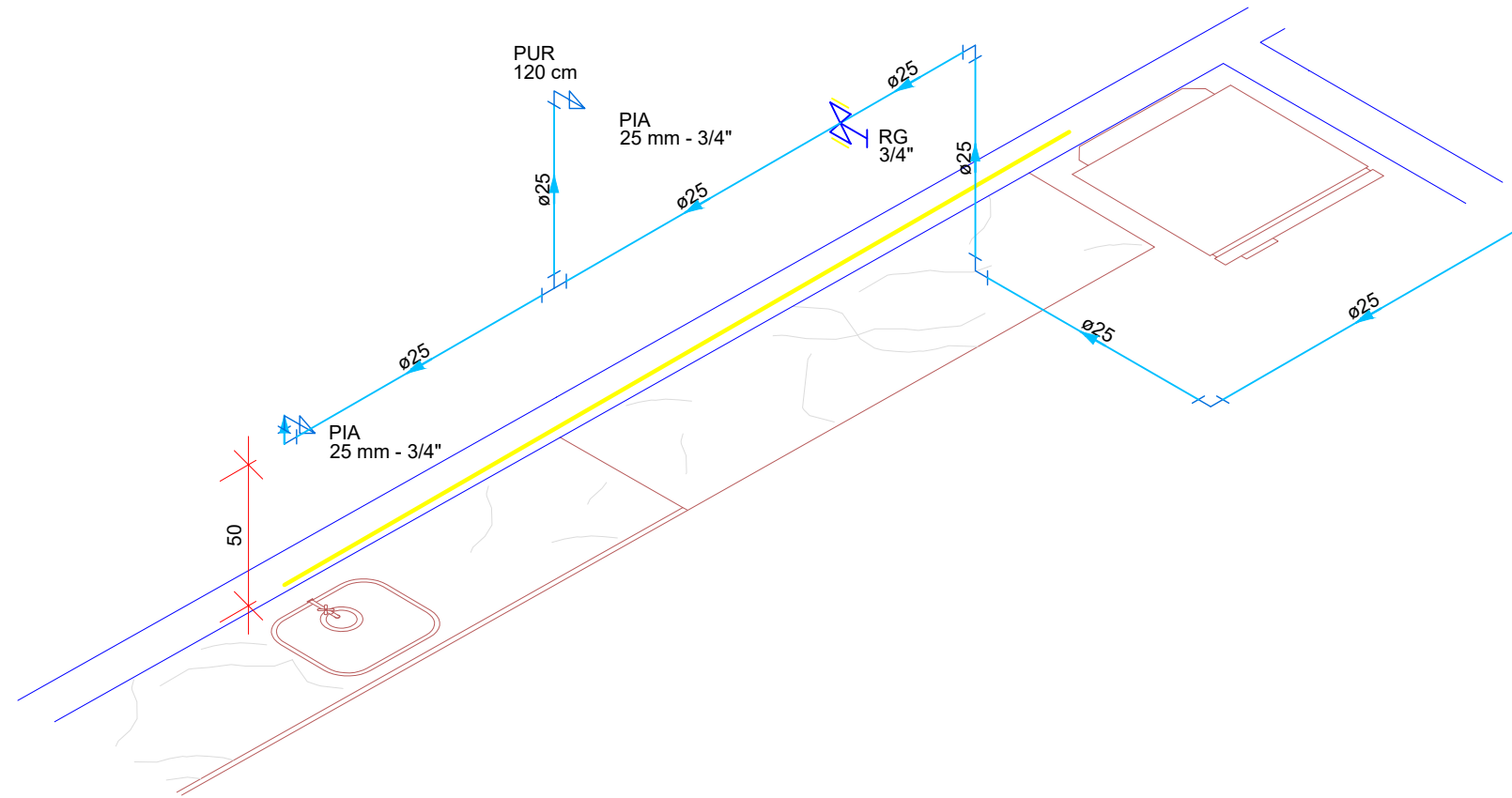
Detalhe HID-1 Escala: 1/25
