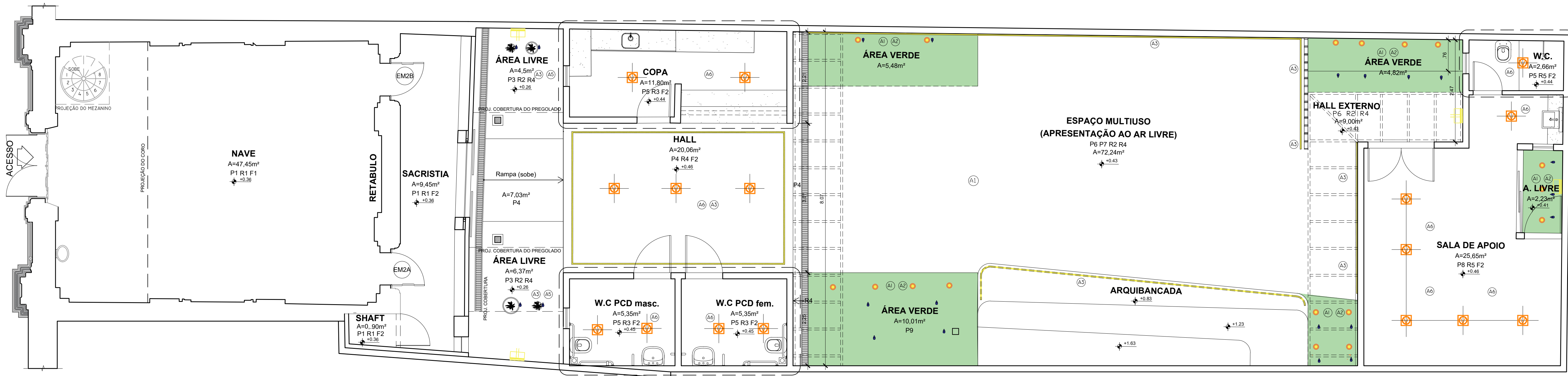
Planta baixa - Luminotécnico
