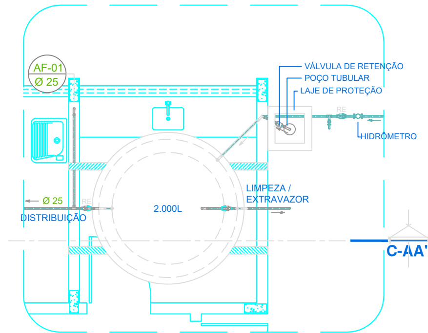
Detalhe Reservatório Elevado escala 1:50
