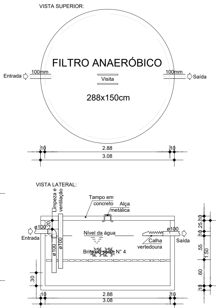
FILTRO ANAERÓBIO TIPO 3 ESC. 1:50
