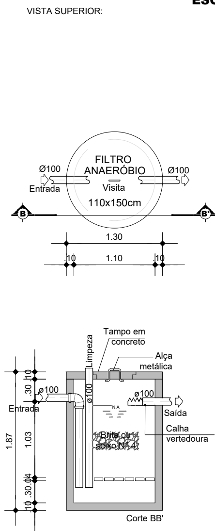
FILTRO ANAERÓBIO TIPO 4 ESC. 1:50
