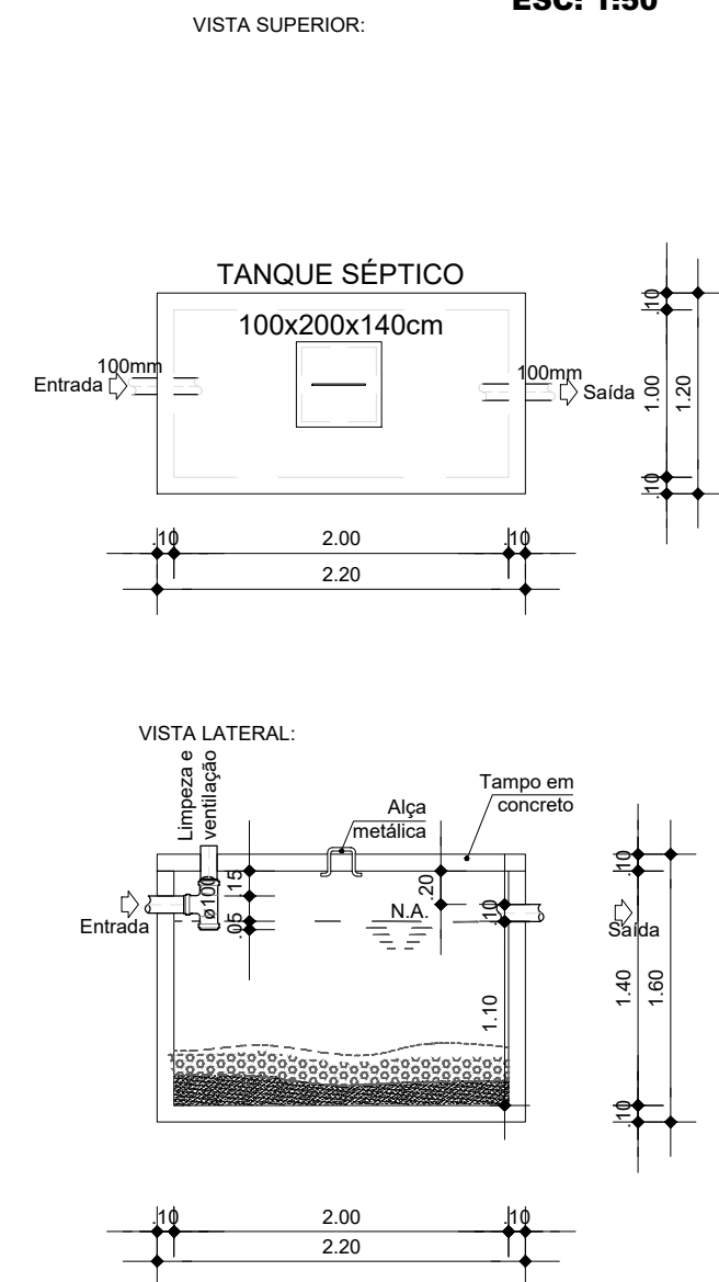
TANQUE SÉPTICO TIPO 4 ESC. 1:50
