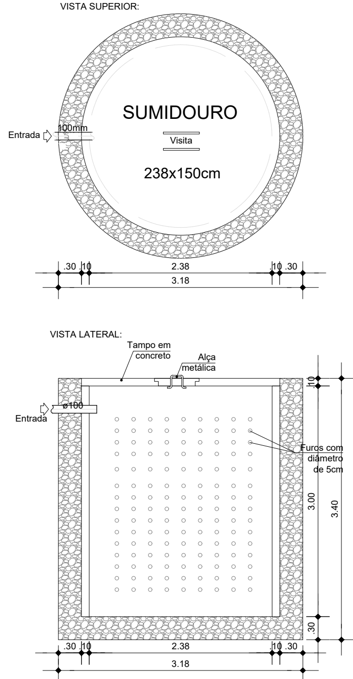
SUMIDOURO TIPO 3 ESC. 1:50
