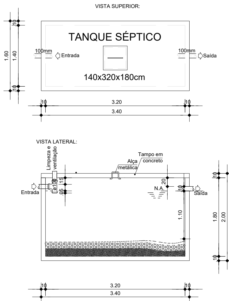
TANQUE SÉPTICO TIPO 3 ESC. 1:50
