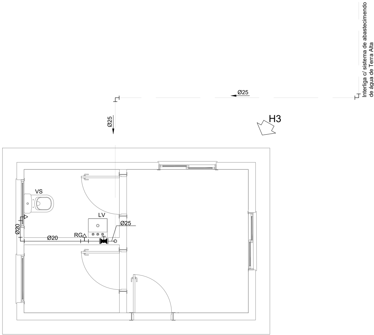
GUARITA INSTALAÇÕES HIDRÁULICAS ESC. 1:50
