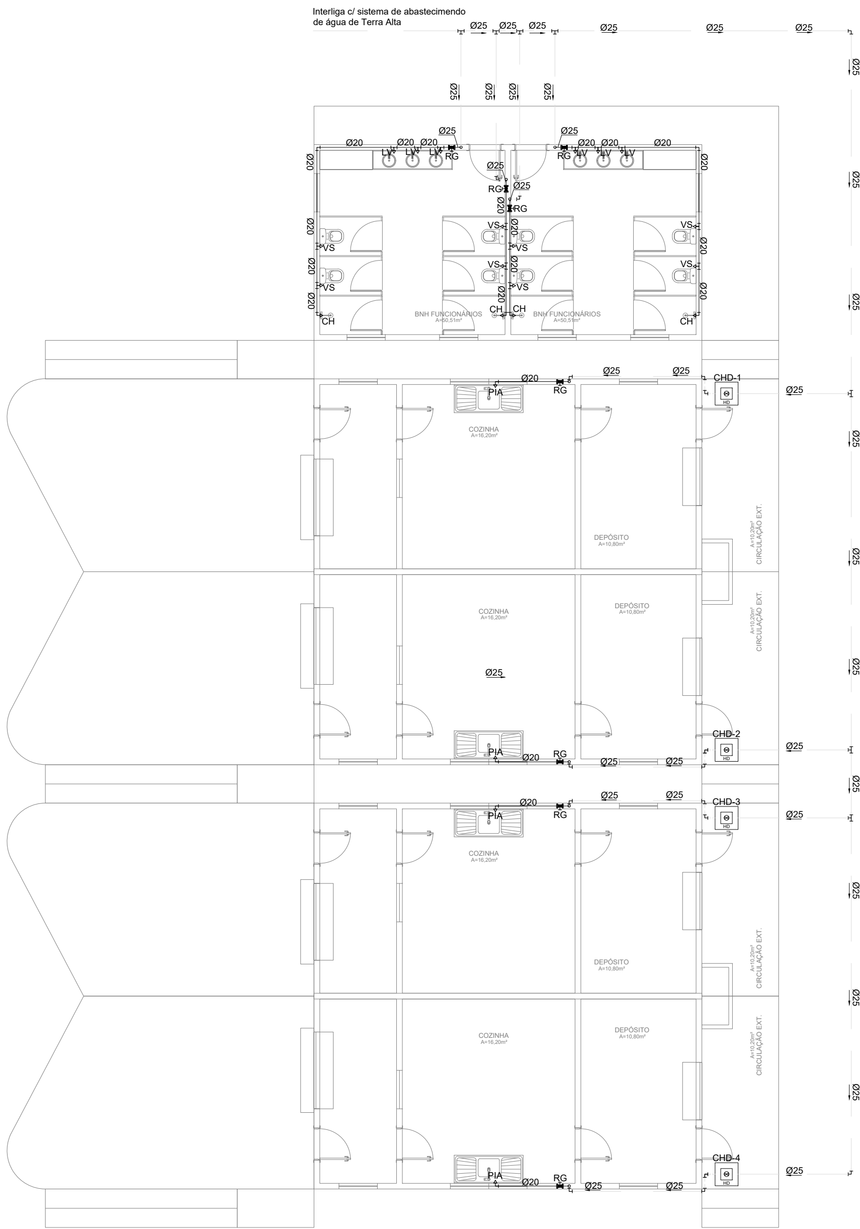
BLOCO B QUIOSQUES INSTALAÇÕES HIDRÁULICAS ESC. 1:100
