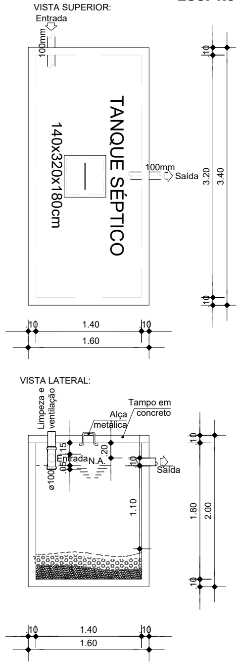
TANQUE SÉPTICO TIPO 2 ESC. 1:50
