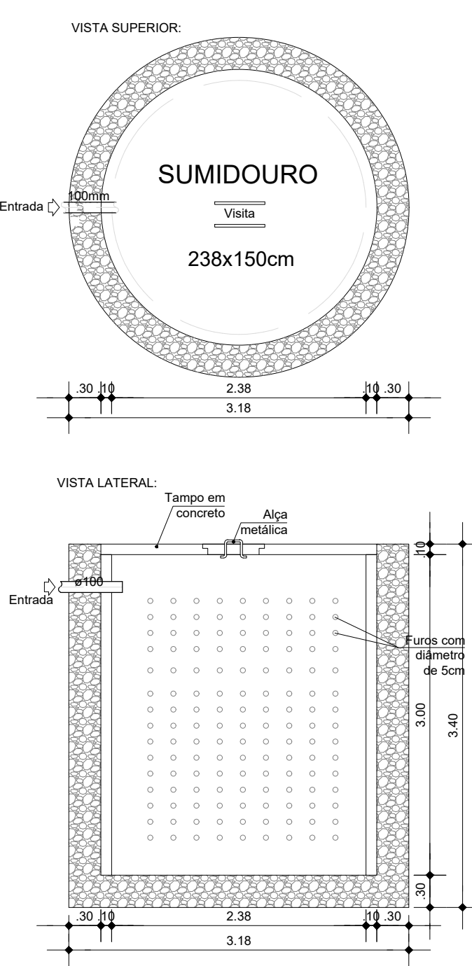
SUMIDOURO TIPO 2 ESC. 1:50
