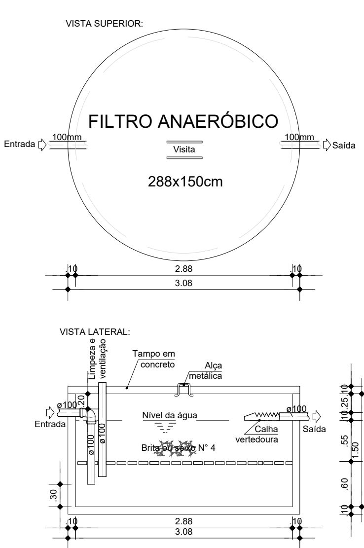
FILTRO ANAERÓBIO TIPO 2 ESC. 1:50
