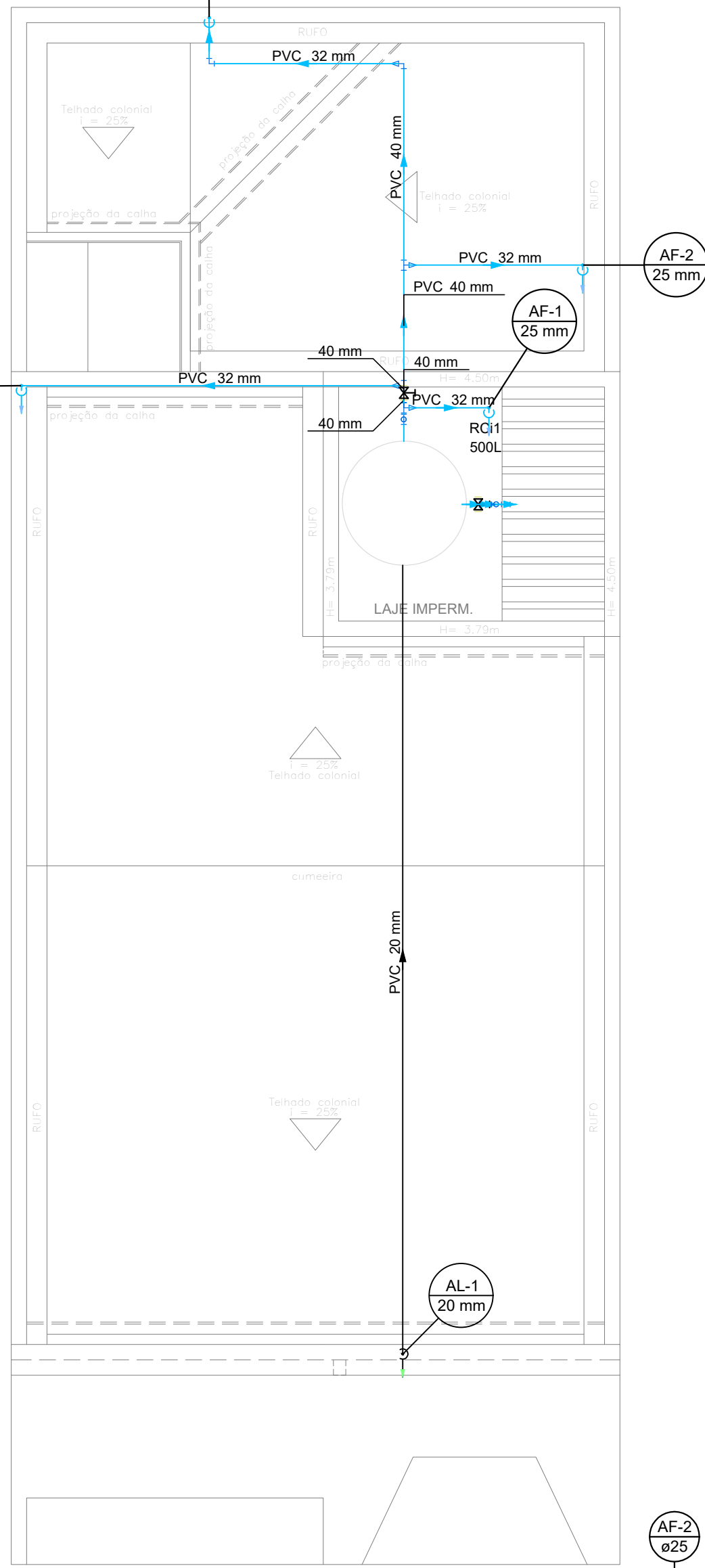
PLANTA BAIXA / COBERTURA ESC.: 1:50
