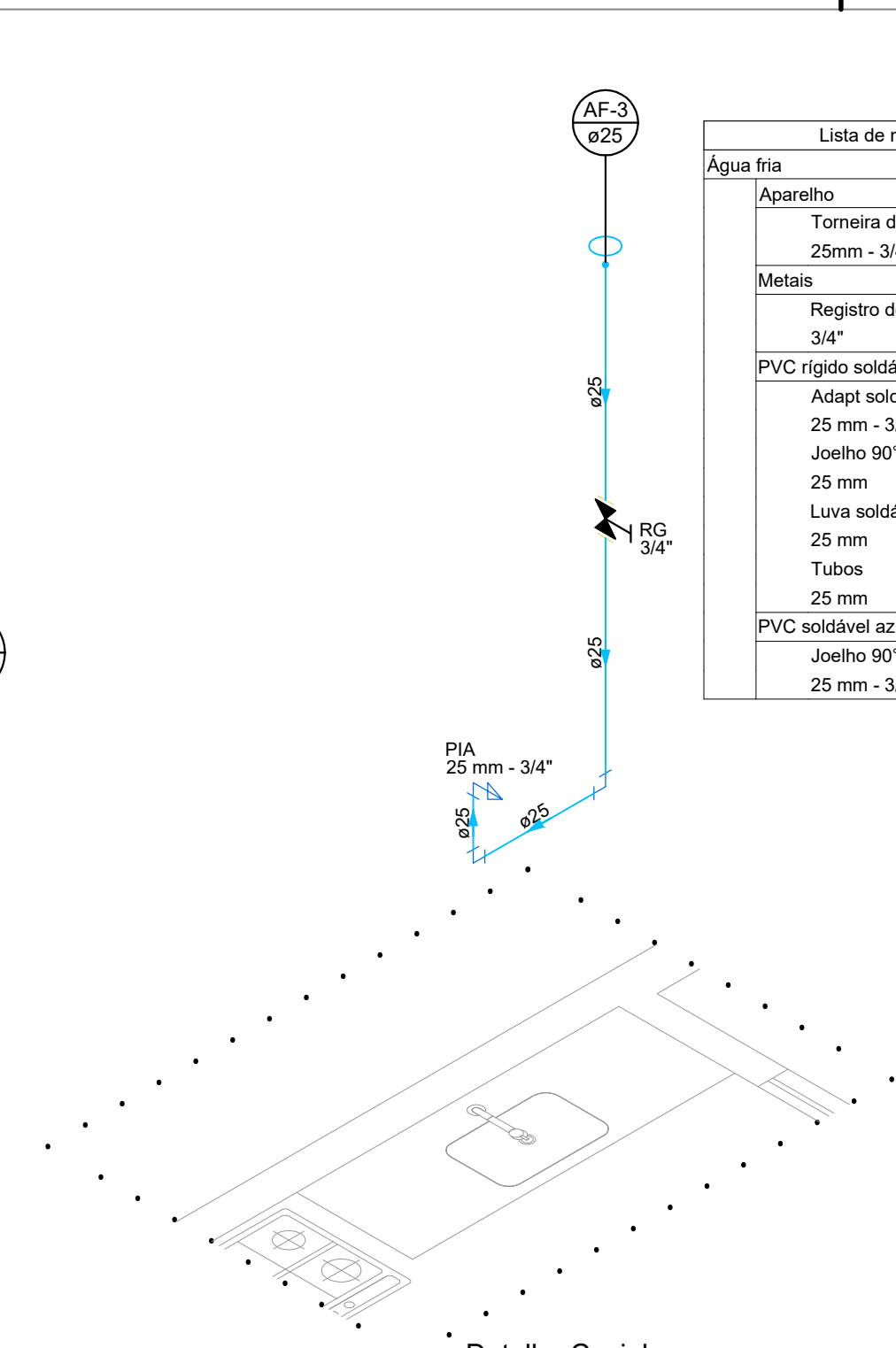
Detalhe Cozinha Escala 1:25
