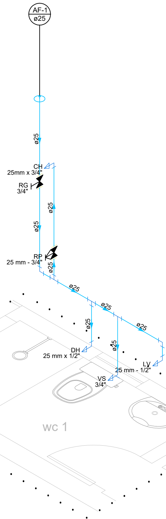
Detalhe WC 1 Escala 1:25
