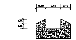
DETALHE DA CALHA VERTEDOURO
