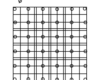
DETALHE DO FUNDO DO FILTRO
