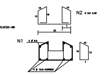
FERRAGEM DA CALHA VERTEDOURO
